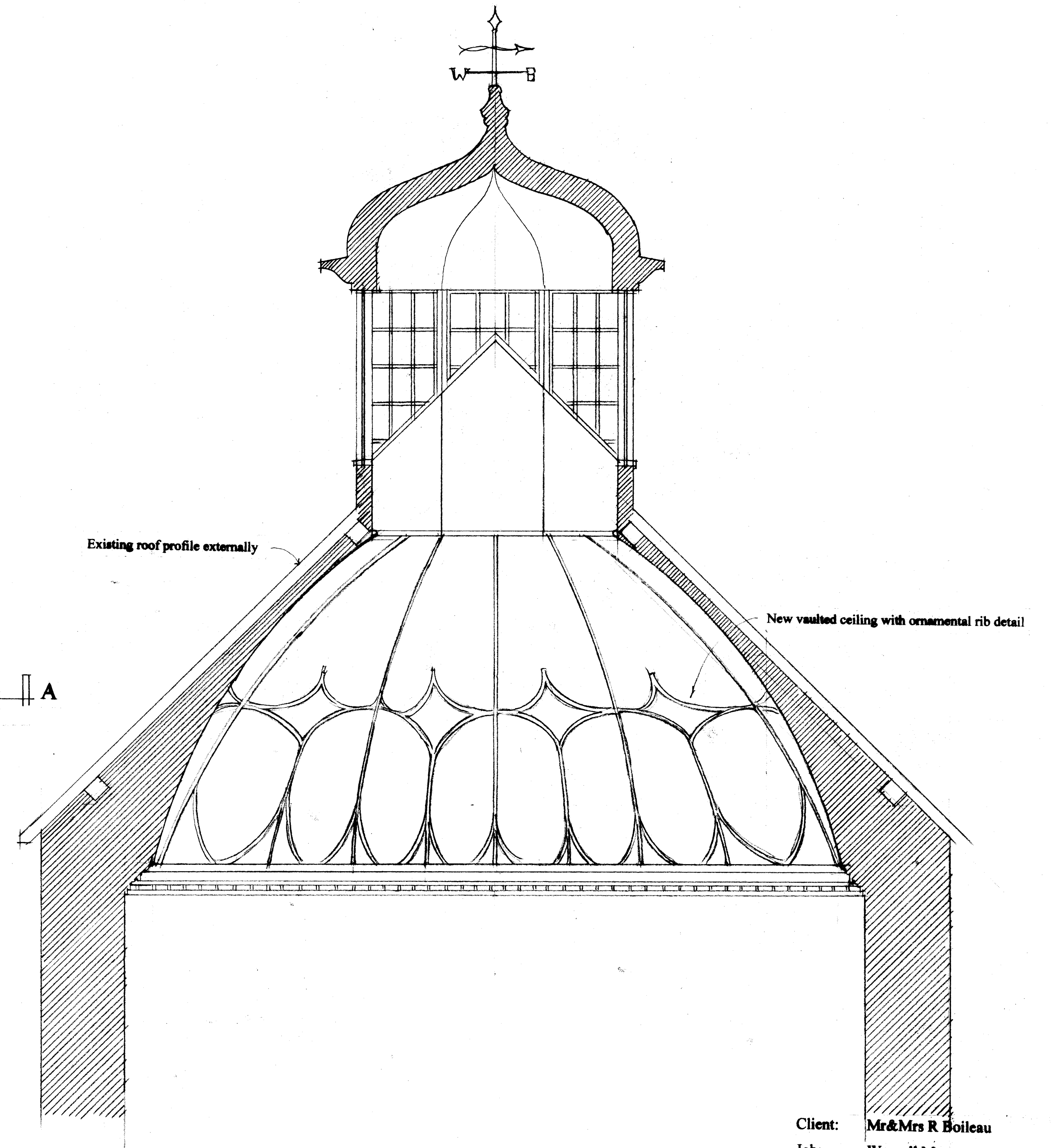
Section A.A. 1:20
