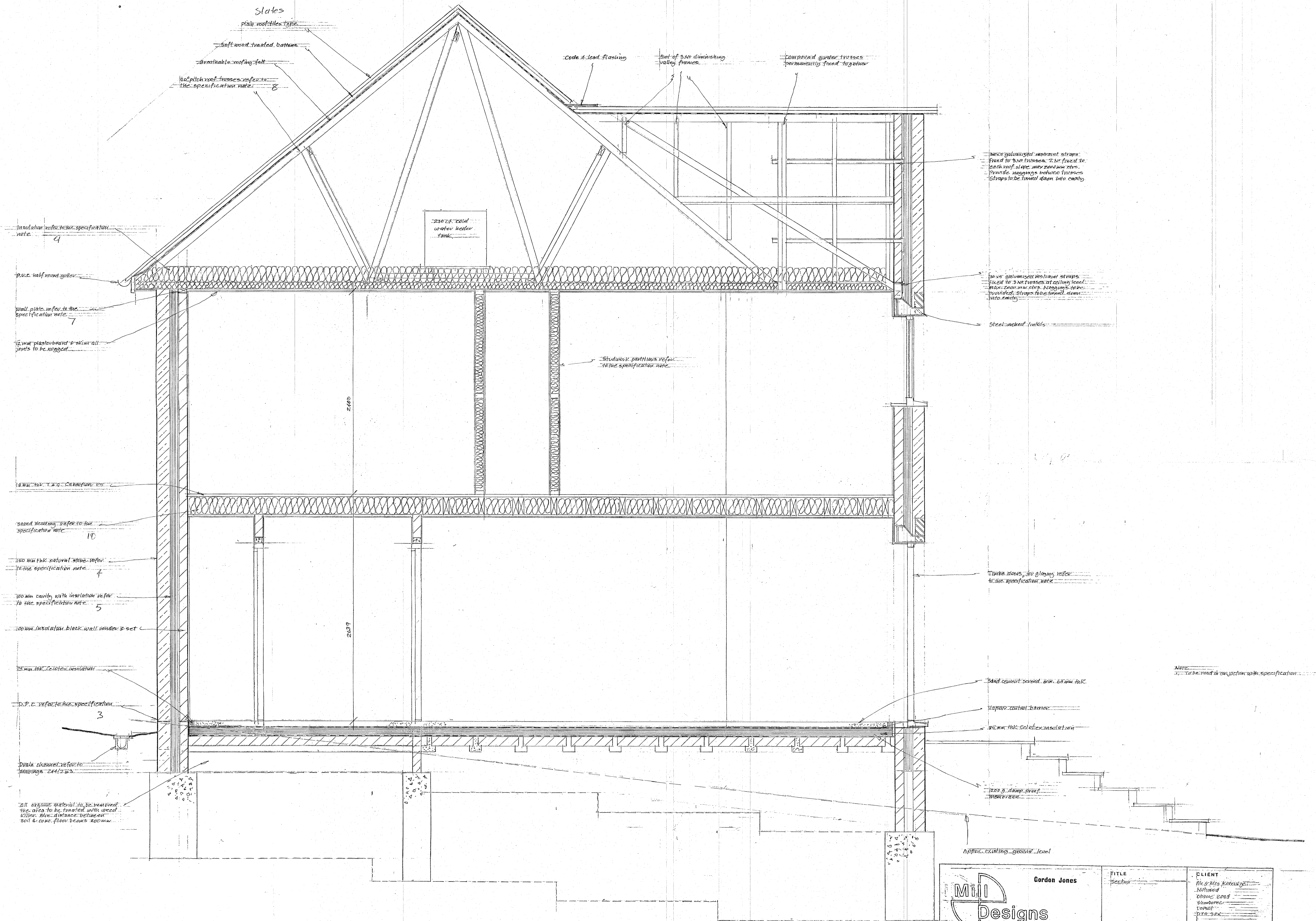
Section d-d
