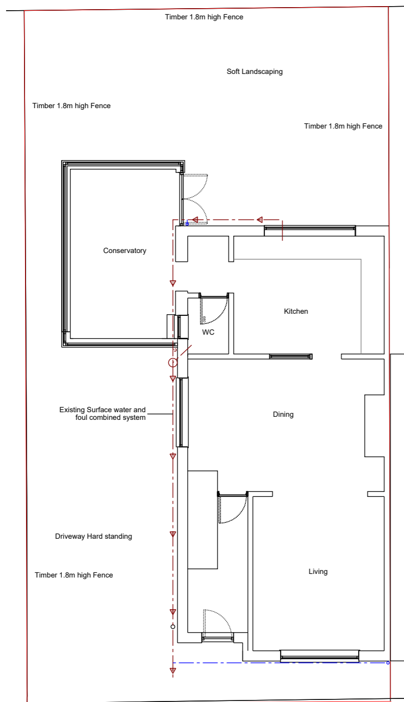
Existing Site Plan 1:100
