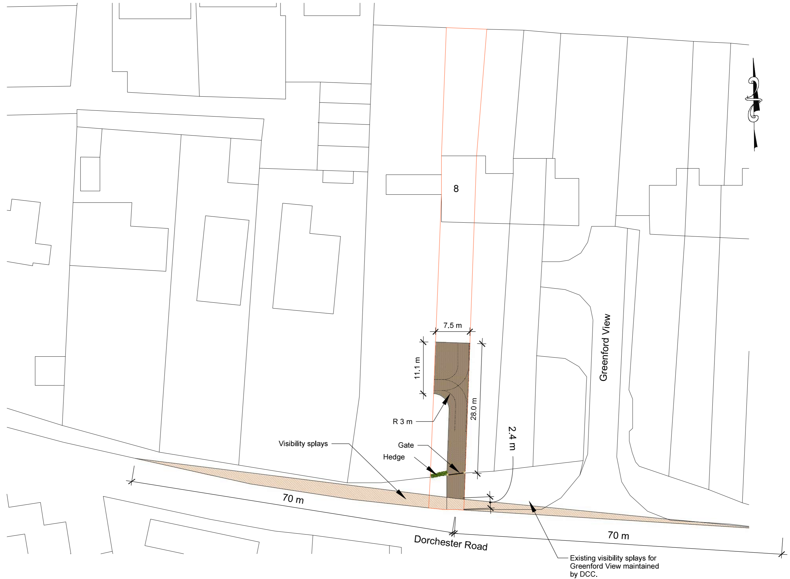
1 Block Plan A02 scale: 1:500
