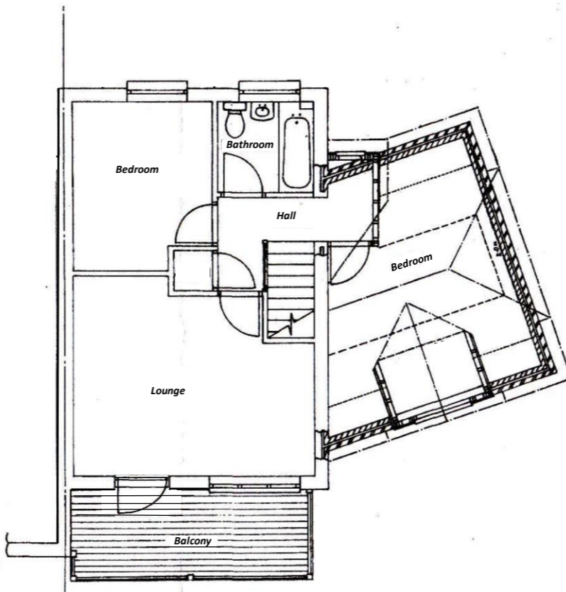
F.F. PLAN.
