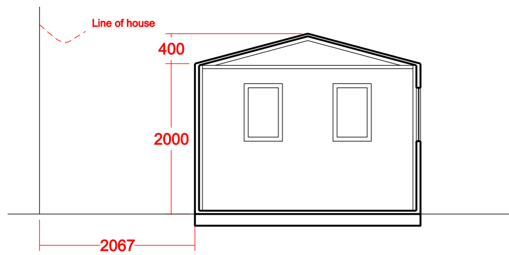
SAA: Section A-A
