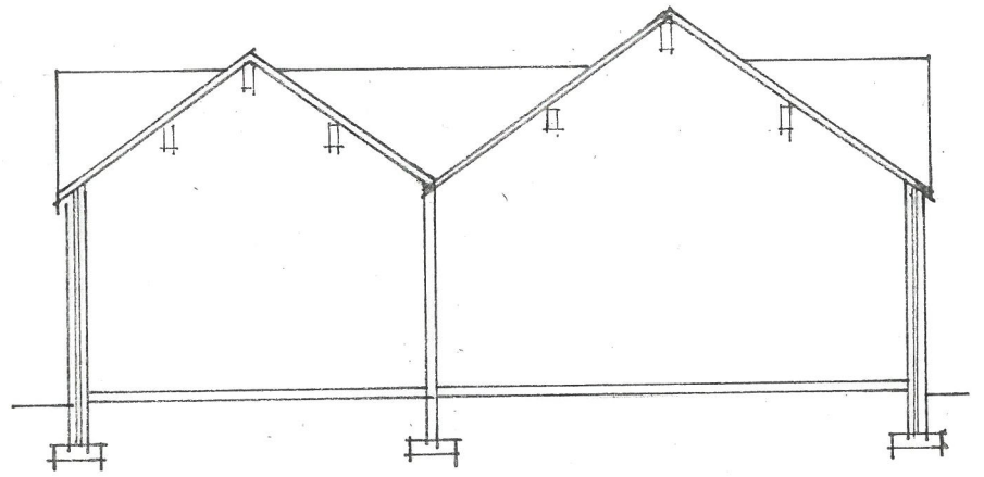
SECTION A-A 1:100
