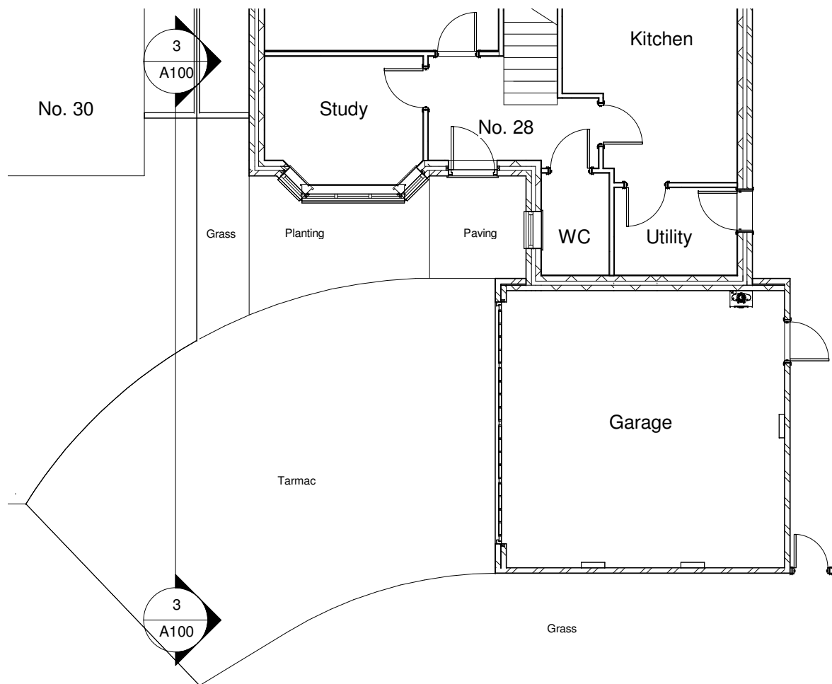
1 Existing Plan 1 : 100
