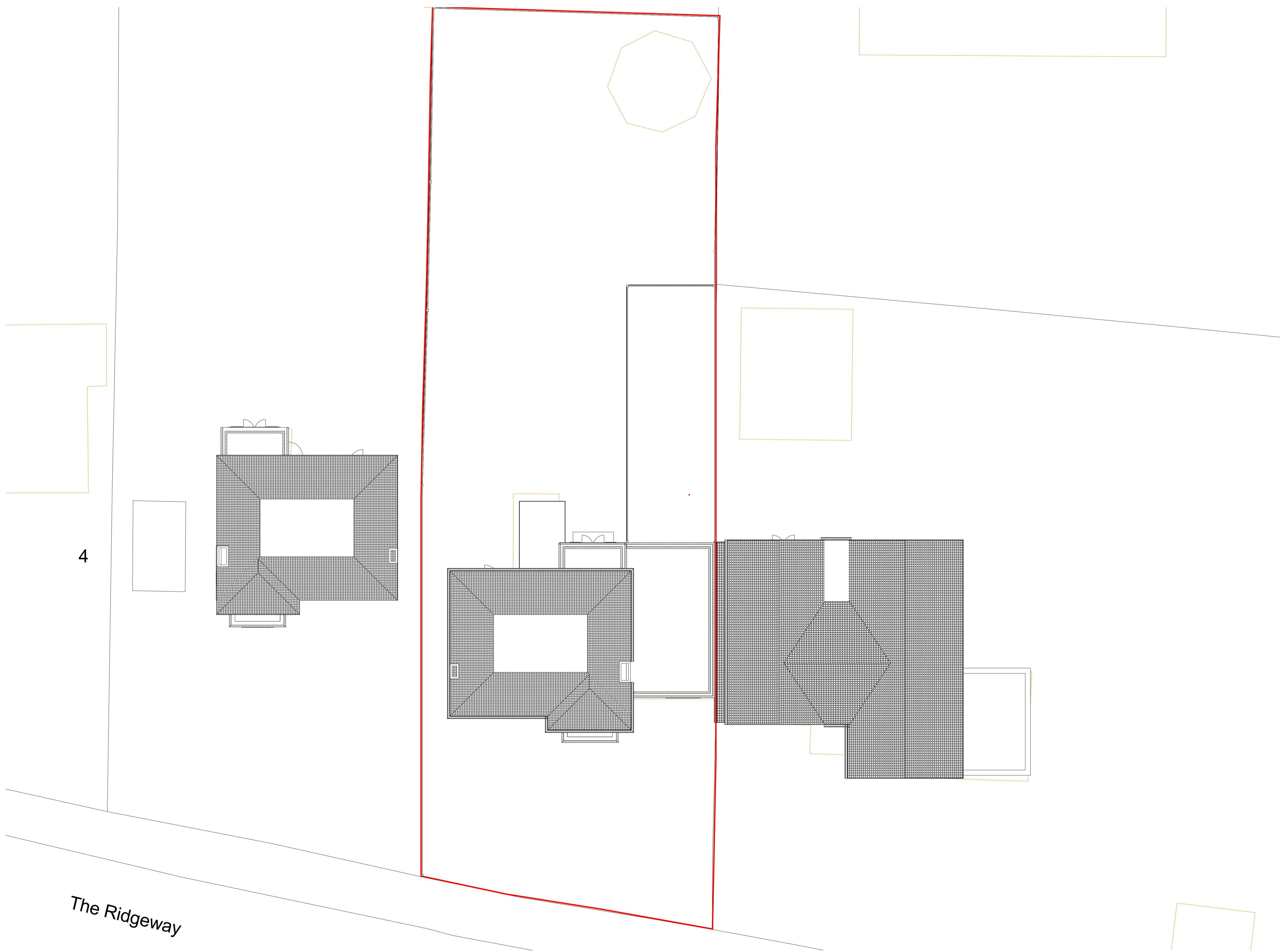
1 Existing Site Plan 1 : 100
