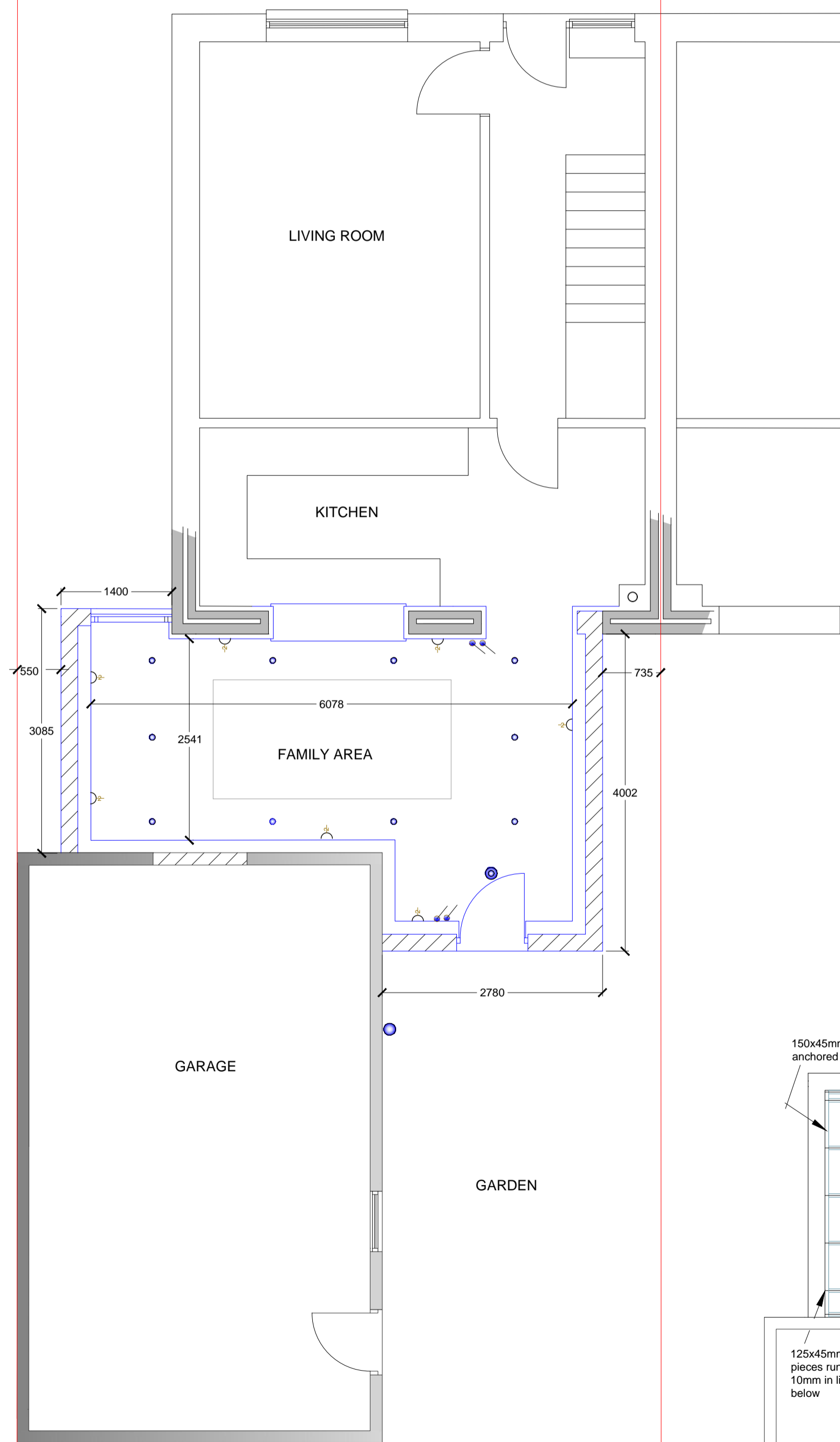
SITE & FLOOR PLAN 1;50
