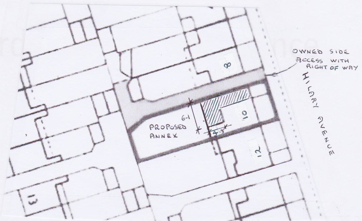
SITE PLAN 1:500
