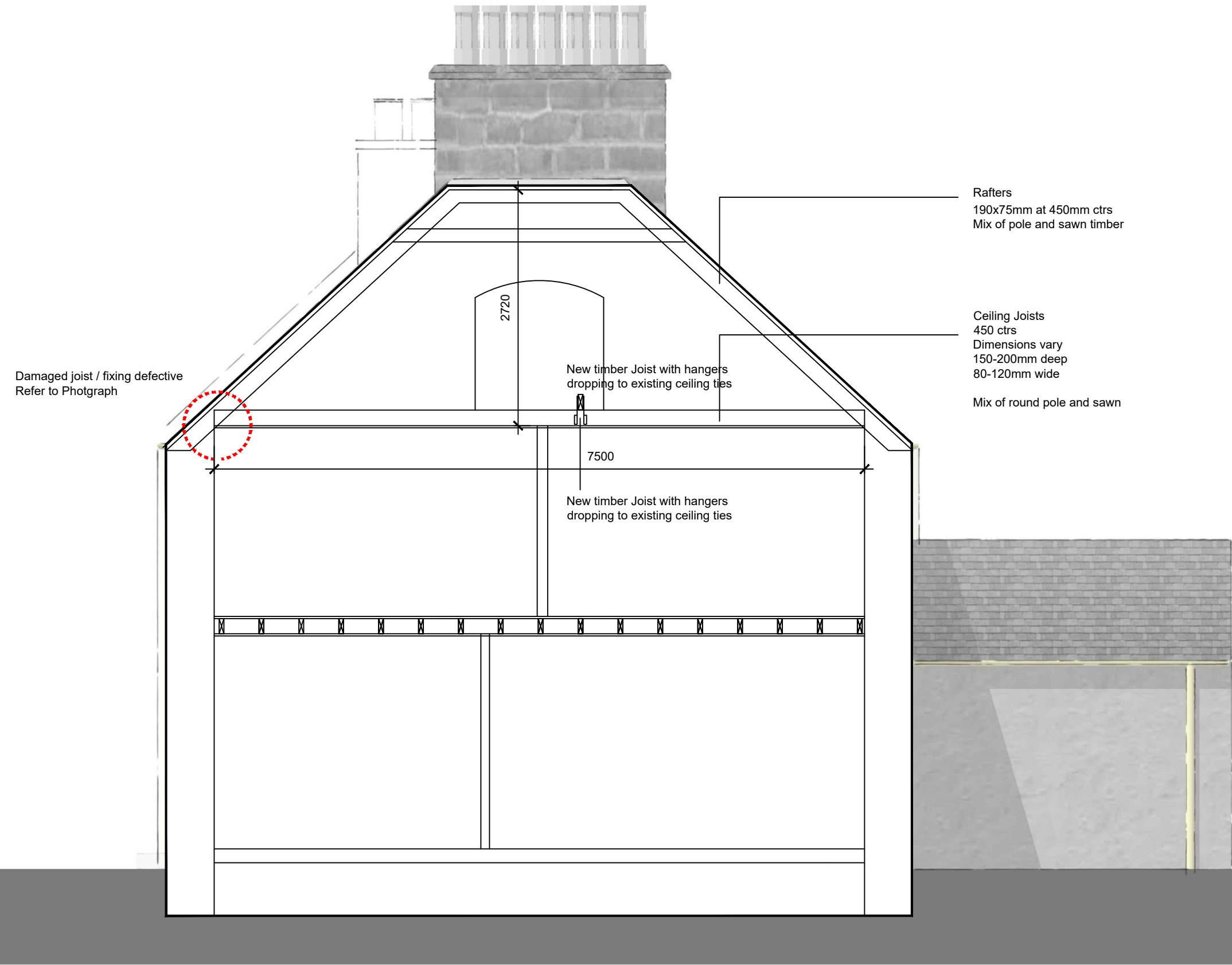
Section - A A3 - 1:50 0 2500mm
