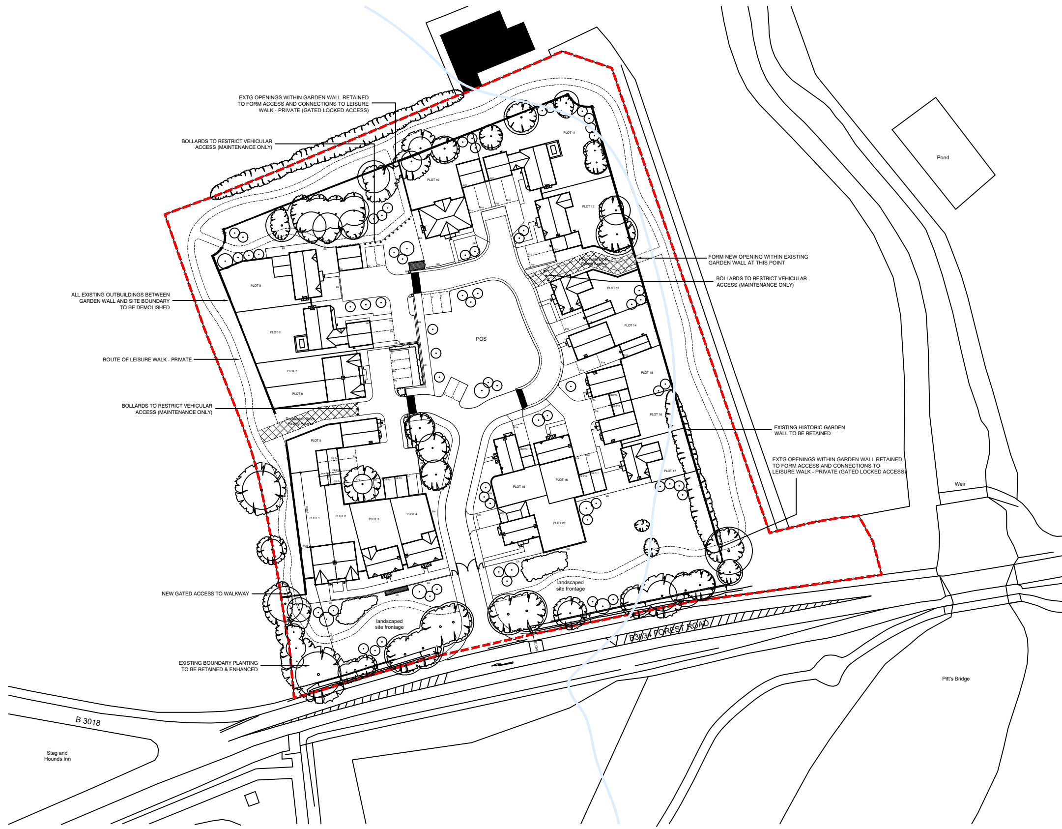
SITE PLAN (1:1000)
