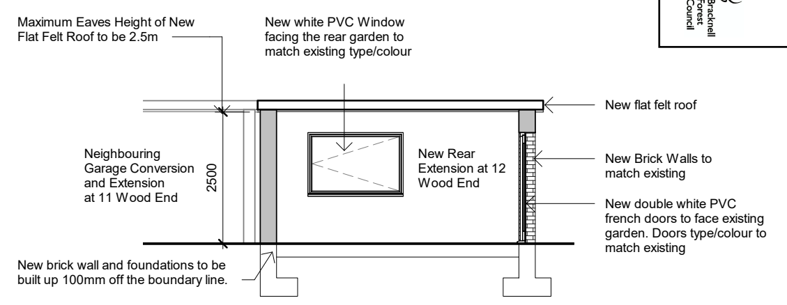
AA SECTION AA 1 : 100
