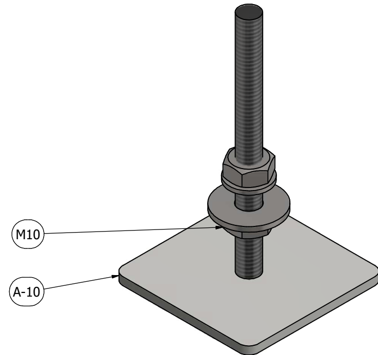
Zestawienie na jedną stopę regulowaną
