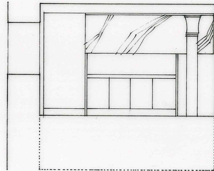
SECTION B.B 1:50
