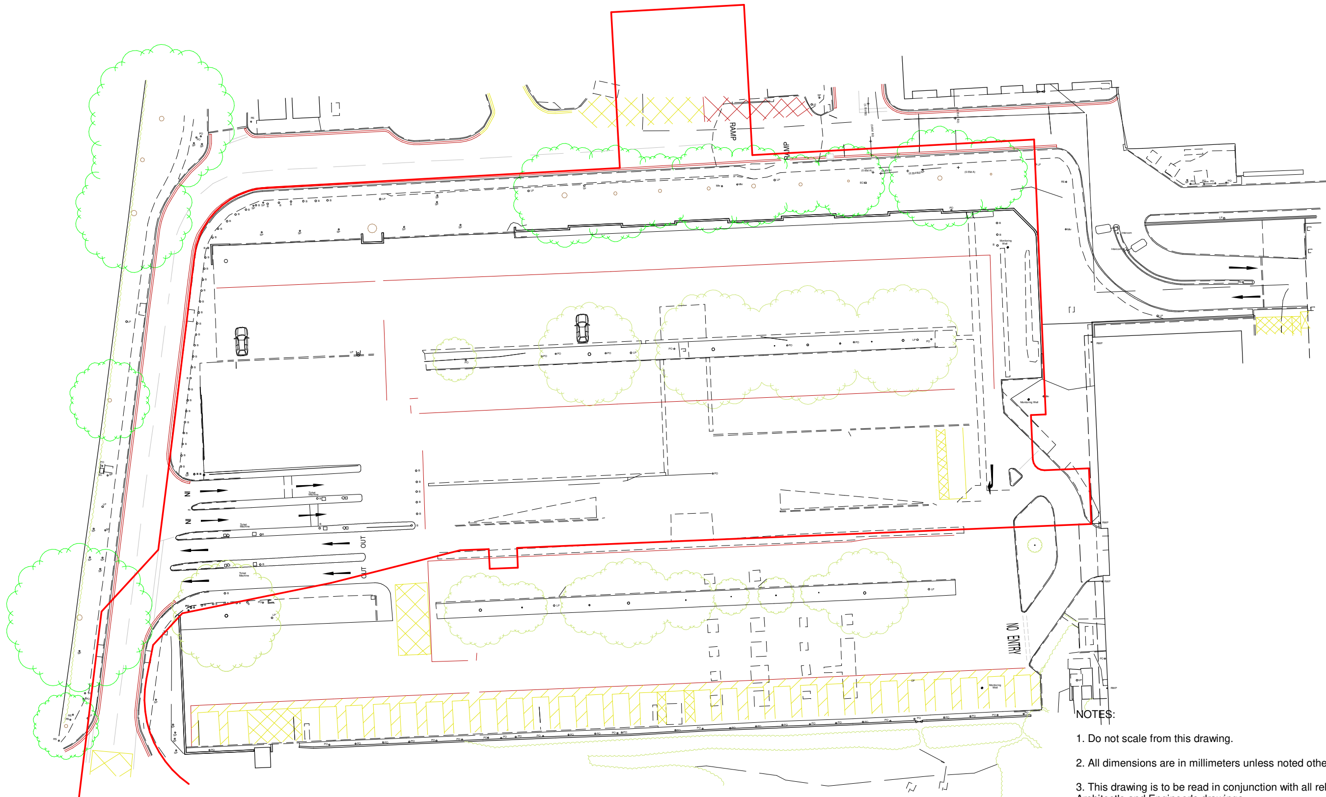
1 Existing site plan 1 : 500
