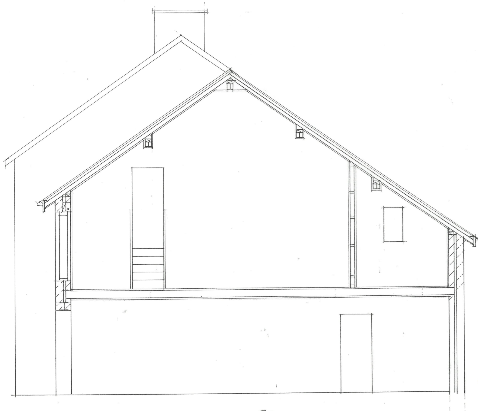
SECTION A-A 1:50
