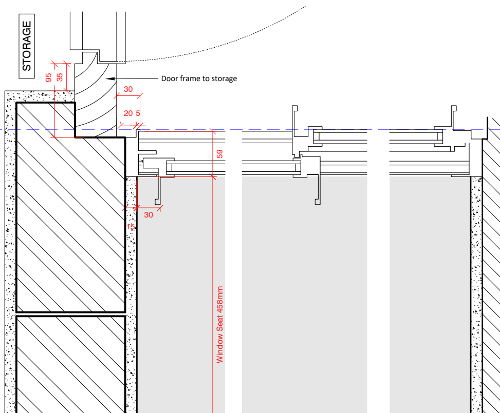
3 Existing Jamb For Type 1a 1:5
