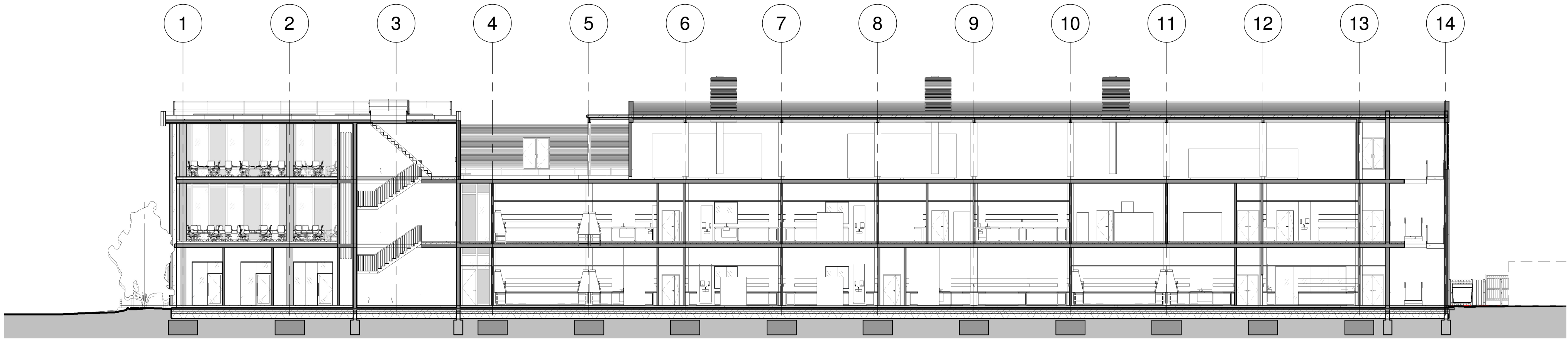
1 Section 1-1 1 : 200
