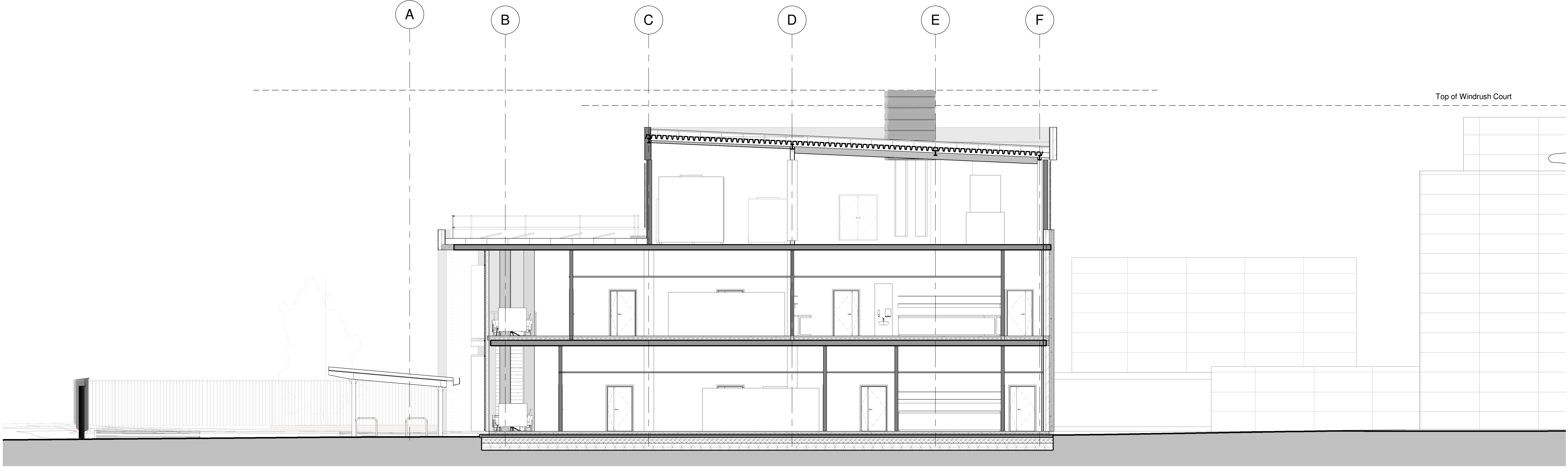
3 Section 3-3 1 : 100
