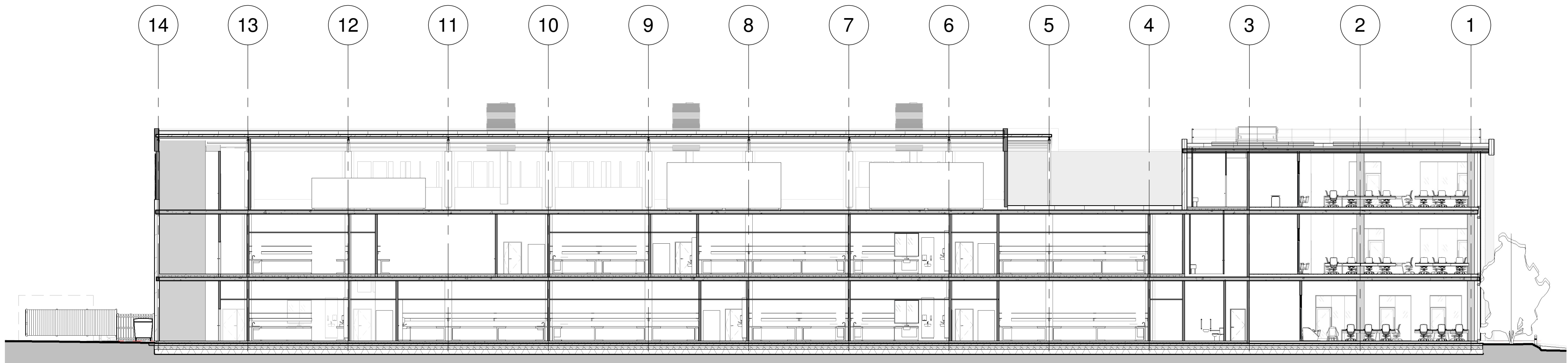
1 Section 1-1 1 : 200
