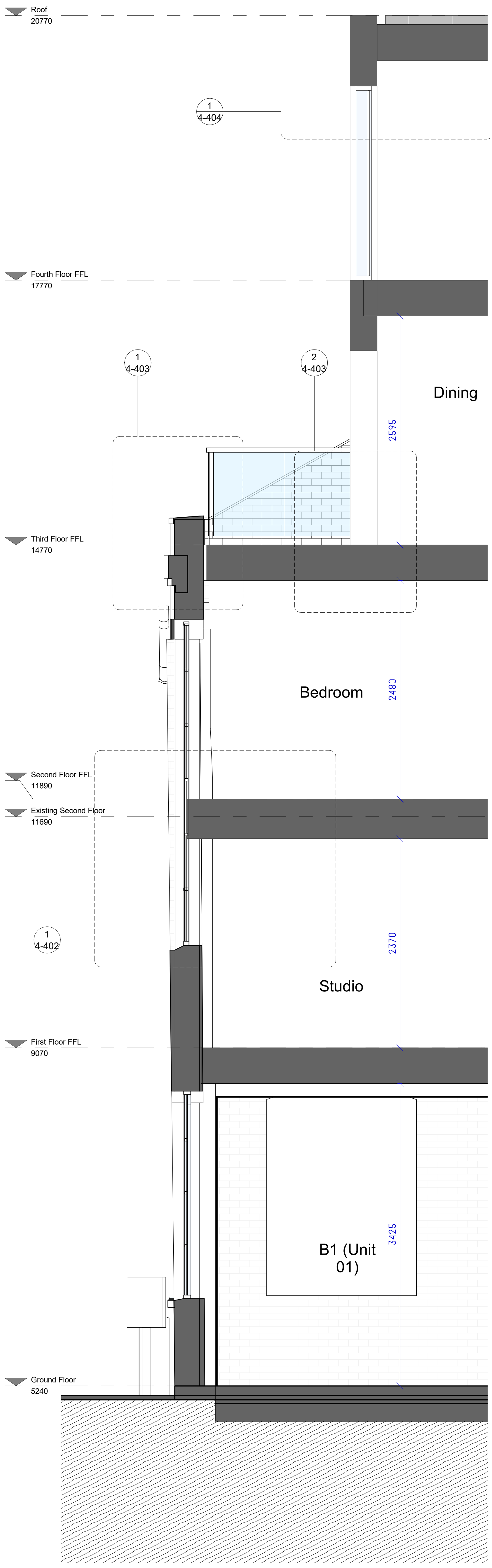
3 Latona Road - Section 1 : 25
