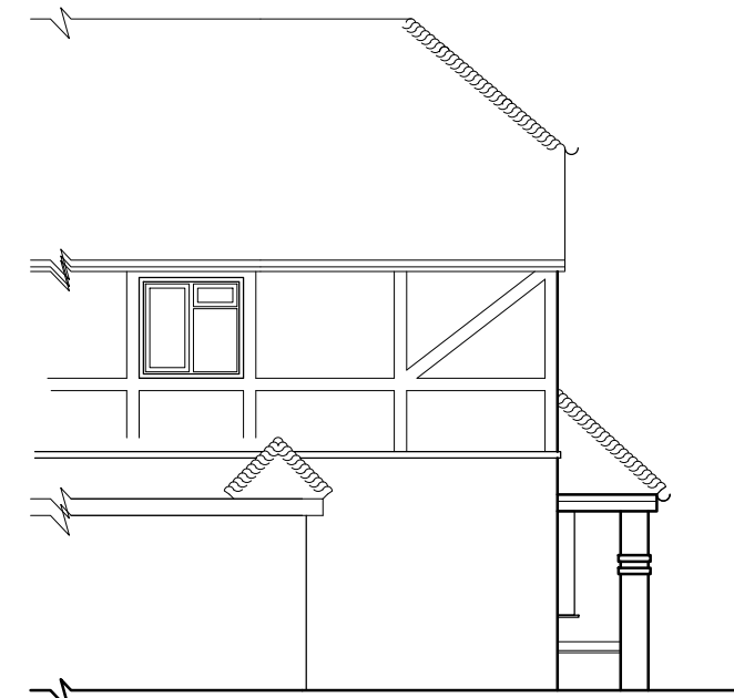
EXISTING SE SIDE ELEVATION
