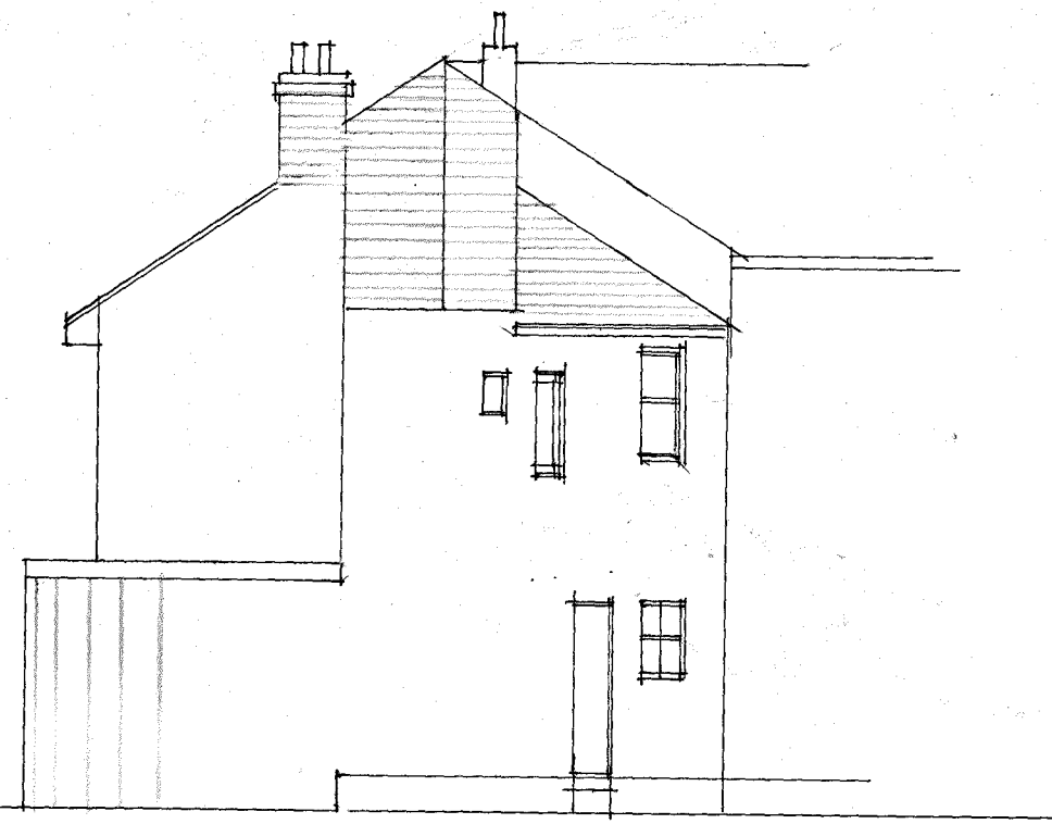
ne elevation
