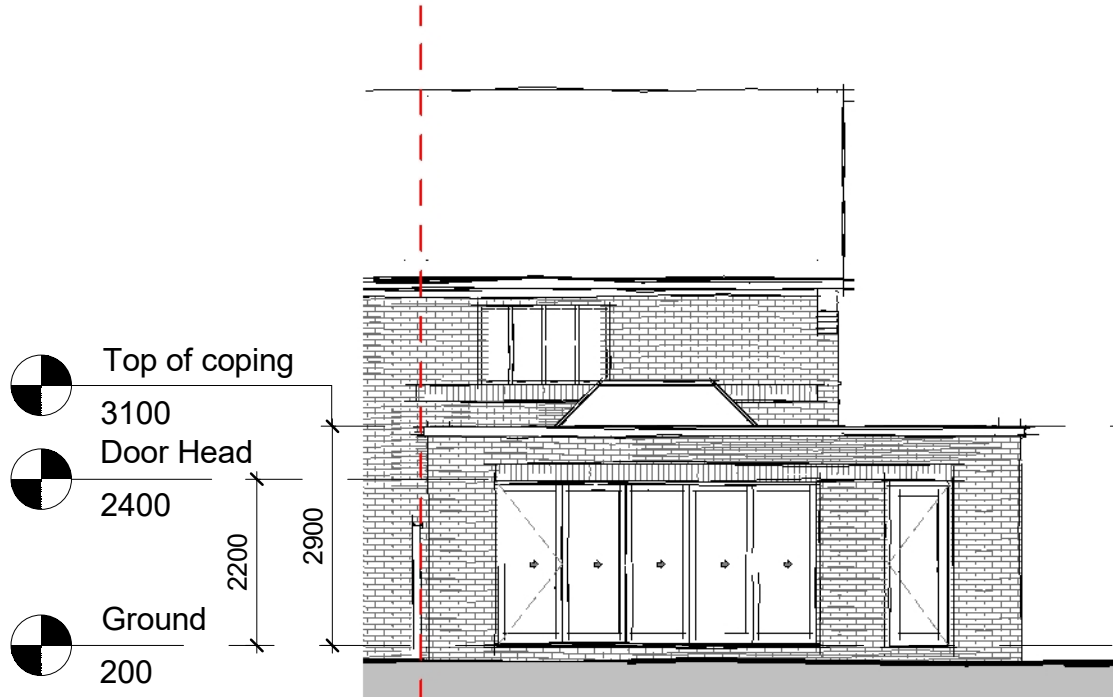
Front 1 : 100
