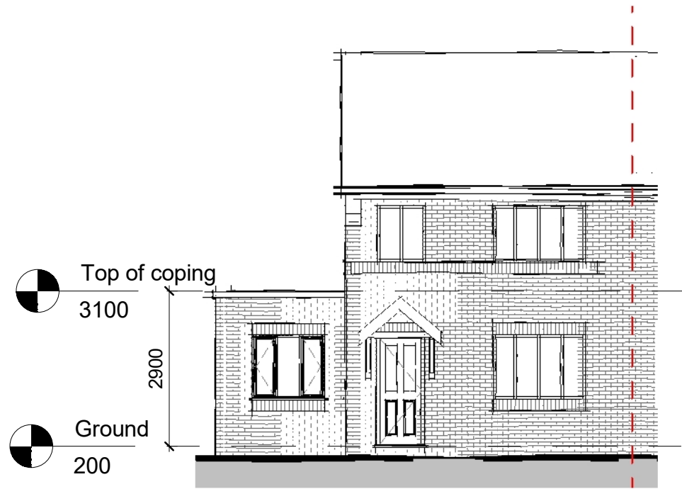
Front 1 : 100
