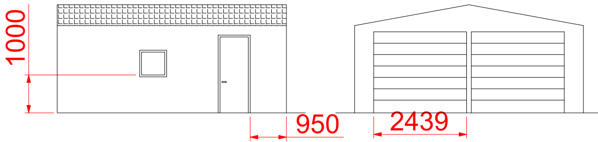
Elevation A
