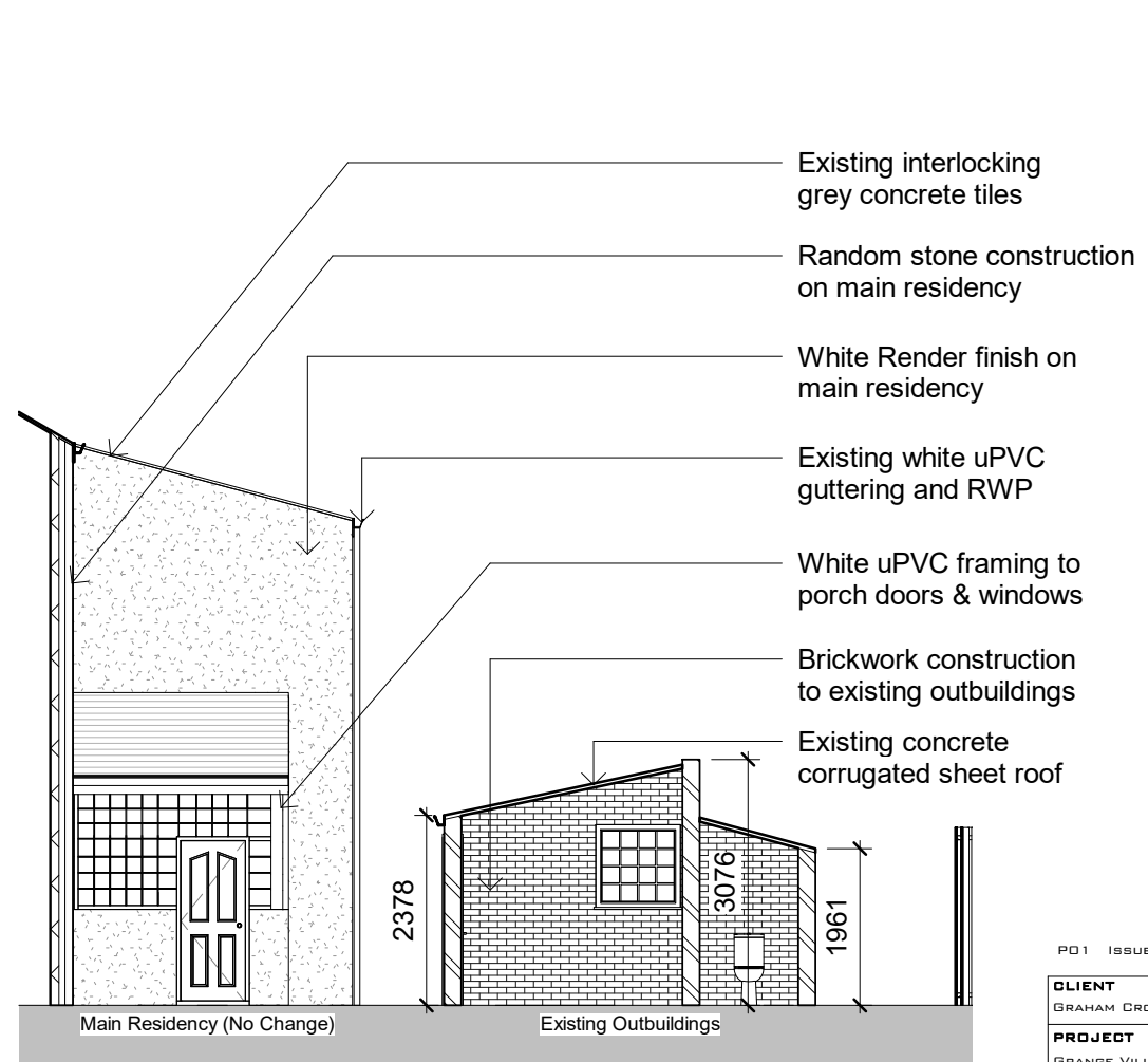
Existing Section AA 1 : 100
