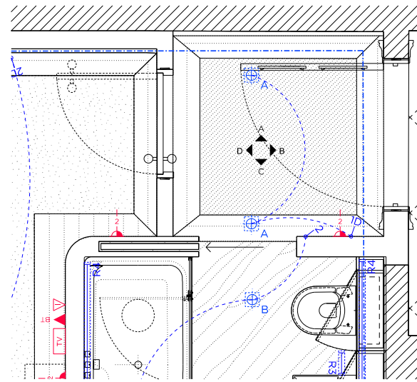
500_001 01 Plan 1:20
