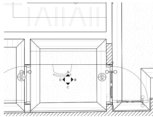
500_004 01 Plan 1:20
