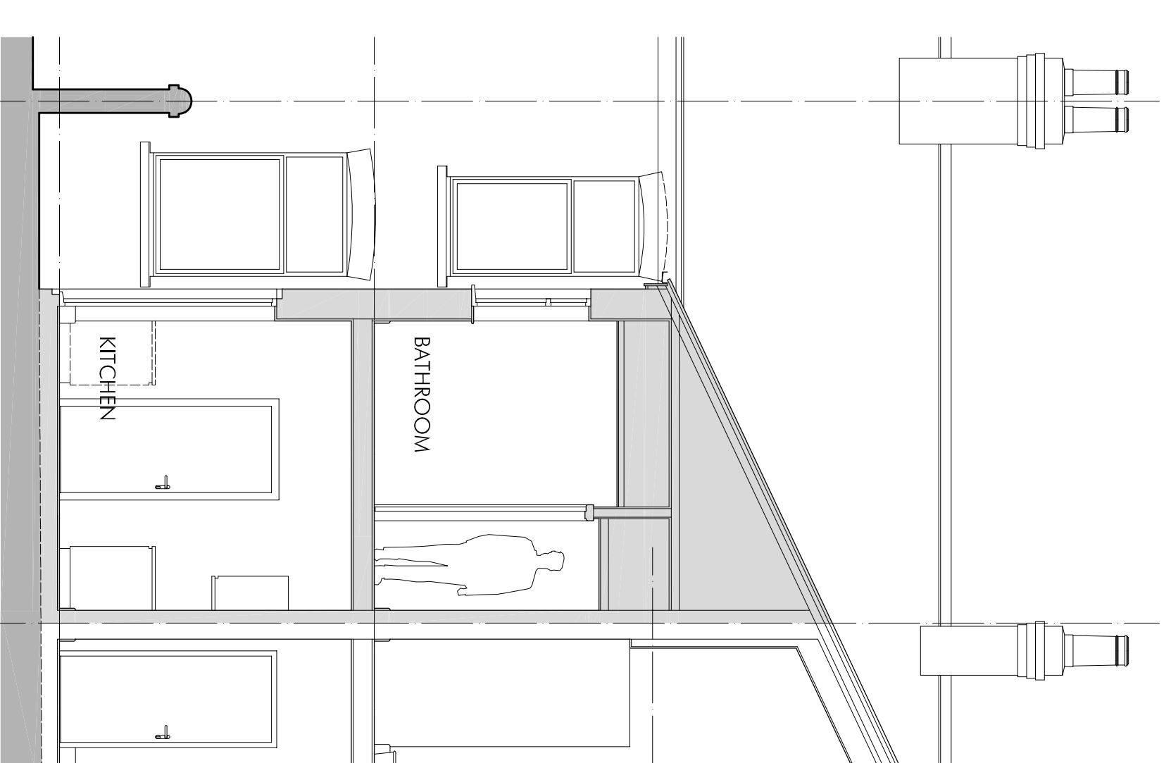
SECTION A-A
