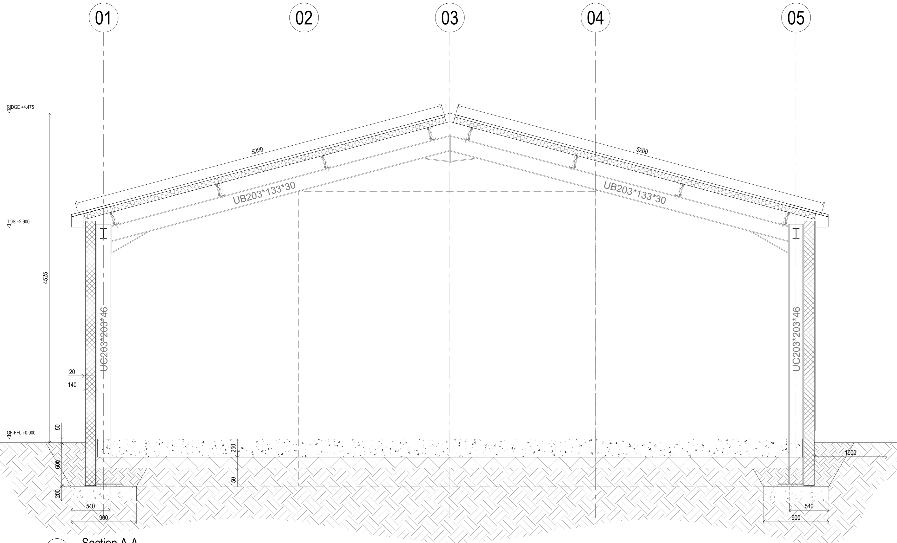
Section A-A Scale: 1:25
