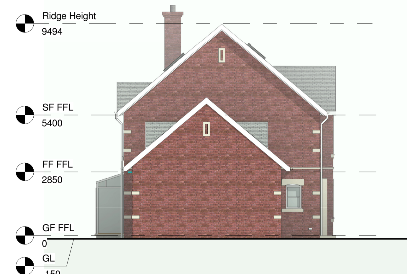
10 West 1 : 100
