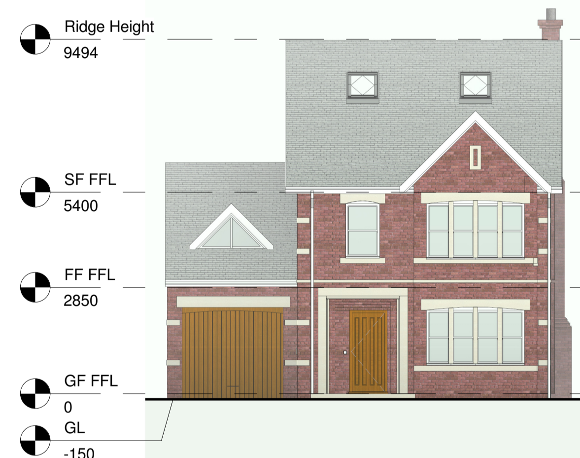
9 South 1 : 100
