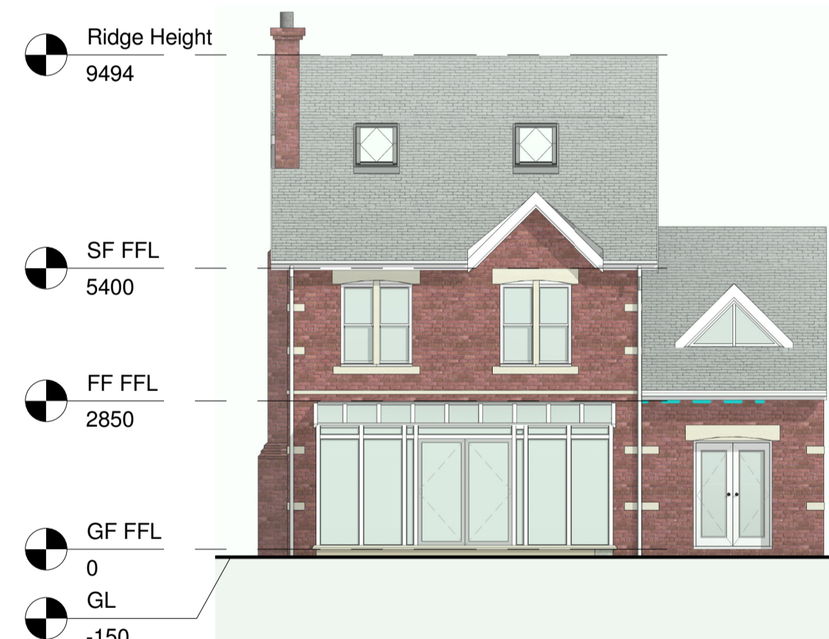
8 North 1 : 100
