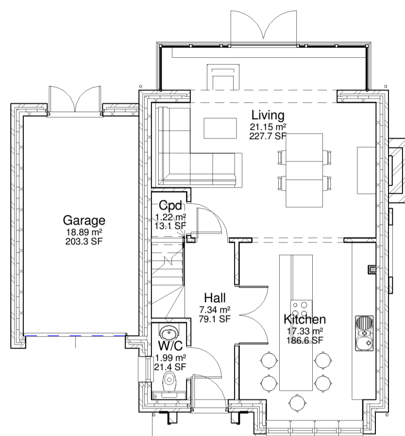
1 GF FFL 1 : 100
