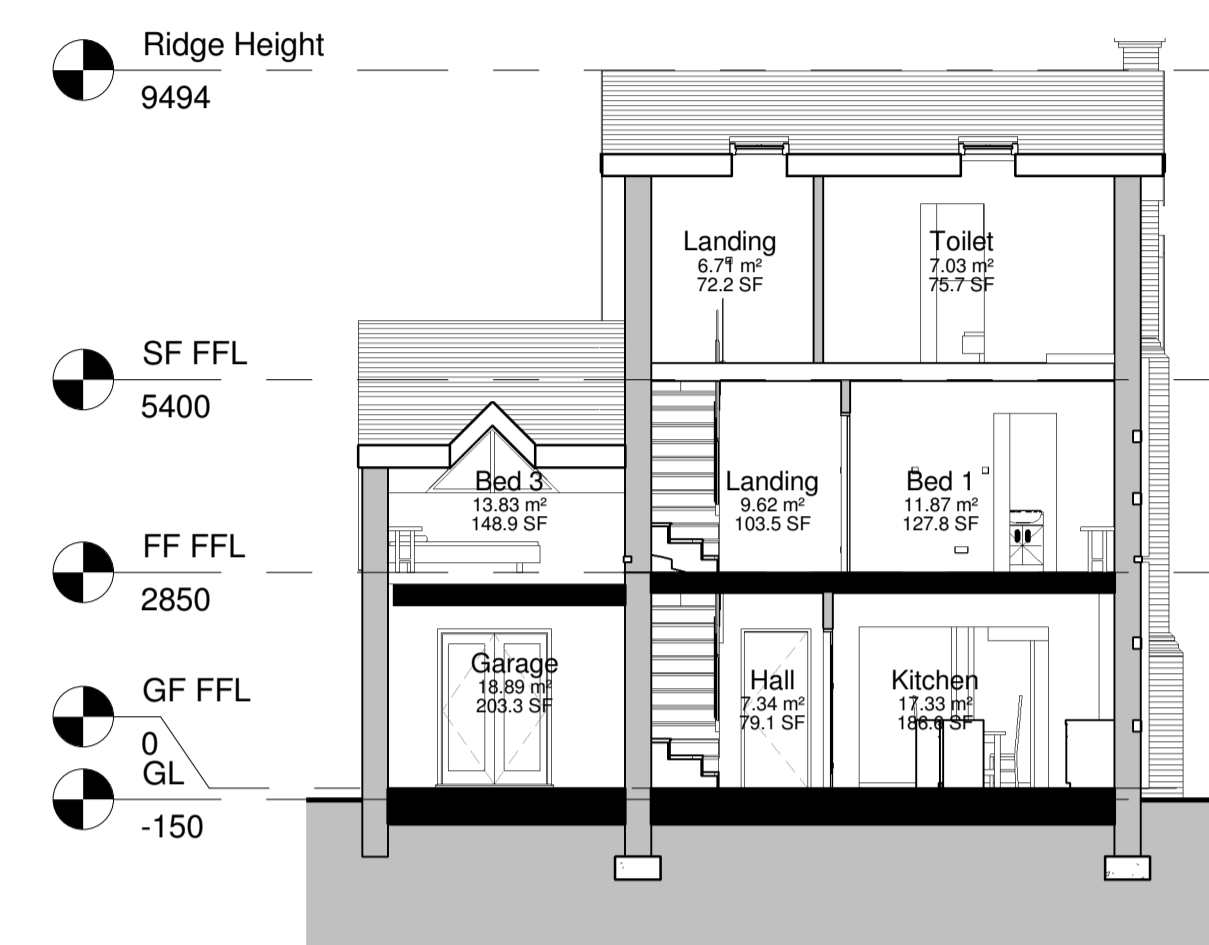
5 Section 1 1 : 100
