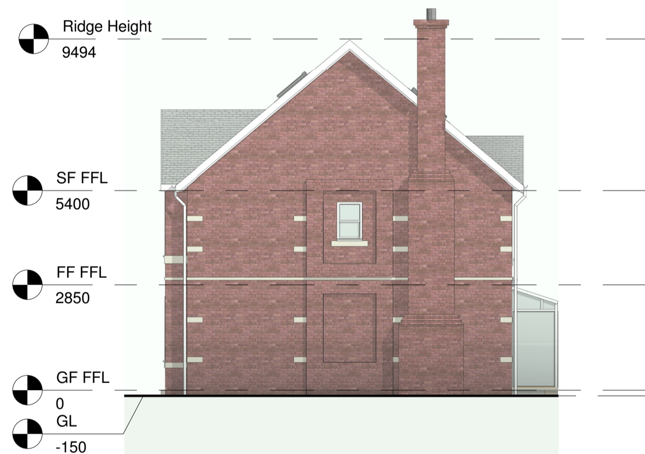
7 East 1 : 100
