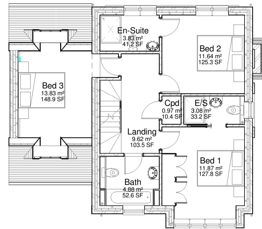
2 FF FFL 1 : 100
