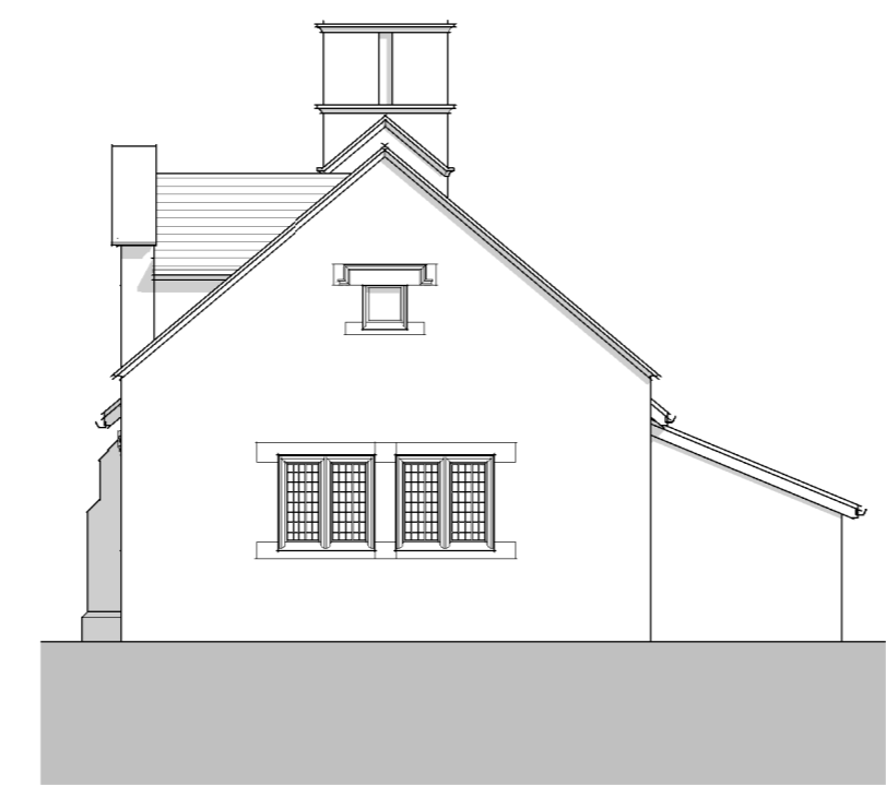
4 Elevation 2 - a 1:100
