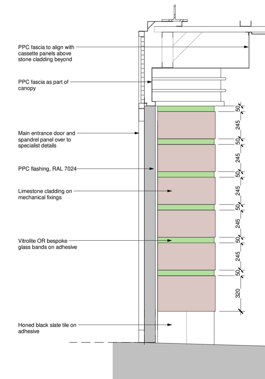
Elev D
