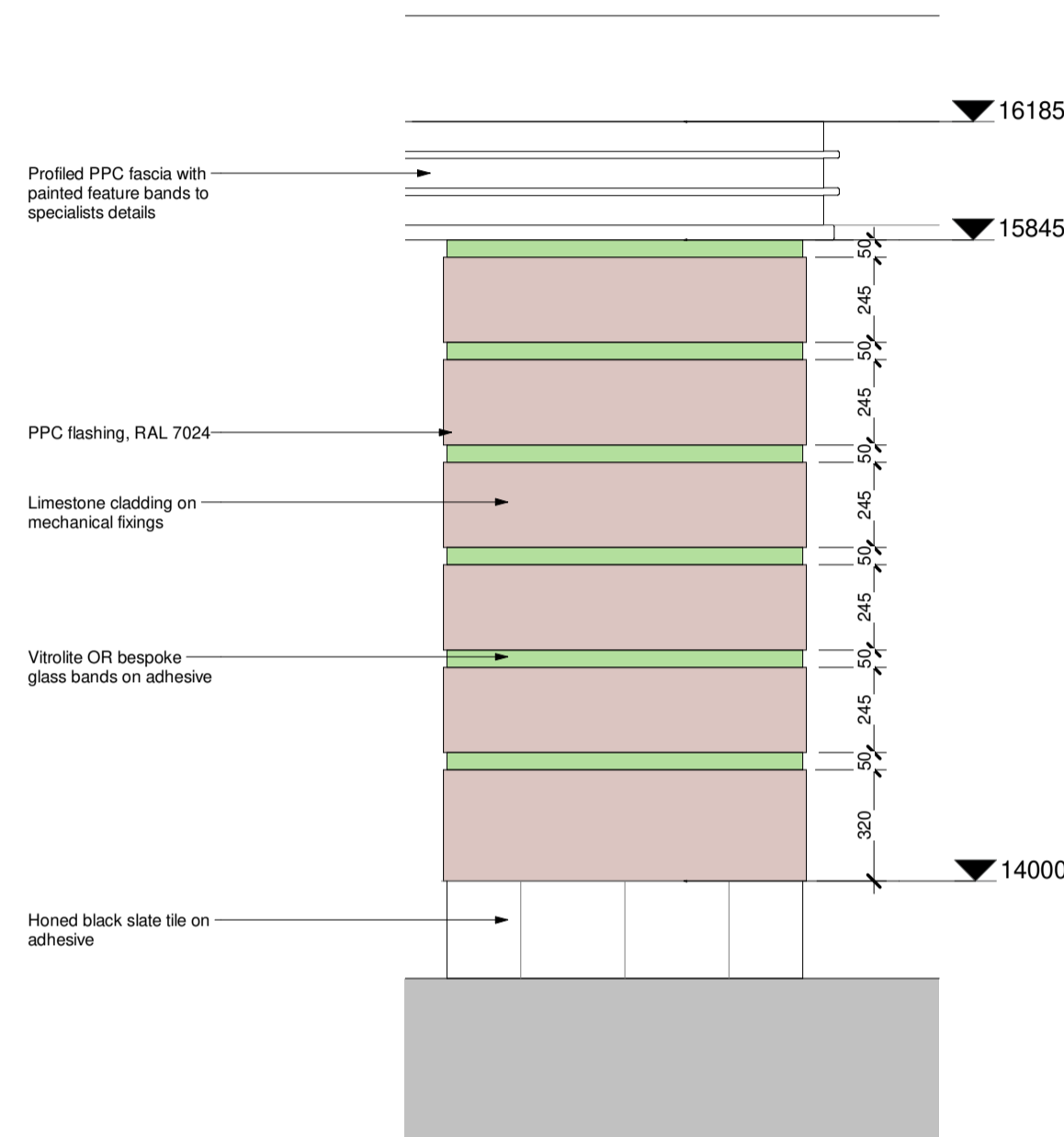
Elev B
