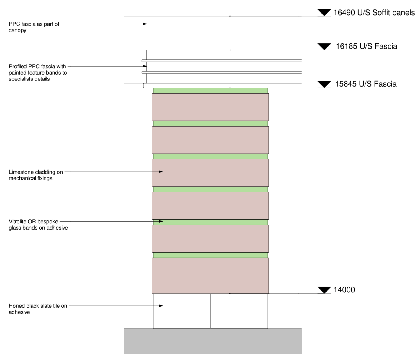
Elev E
