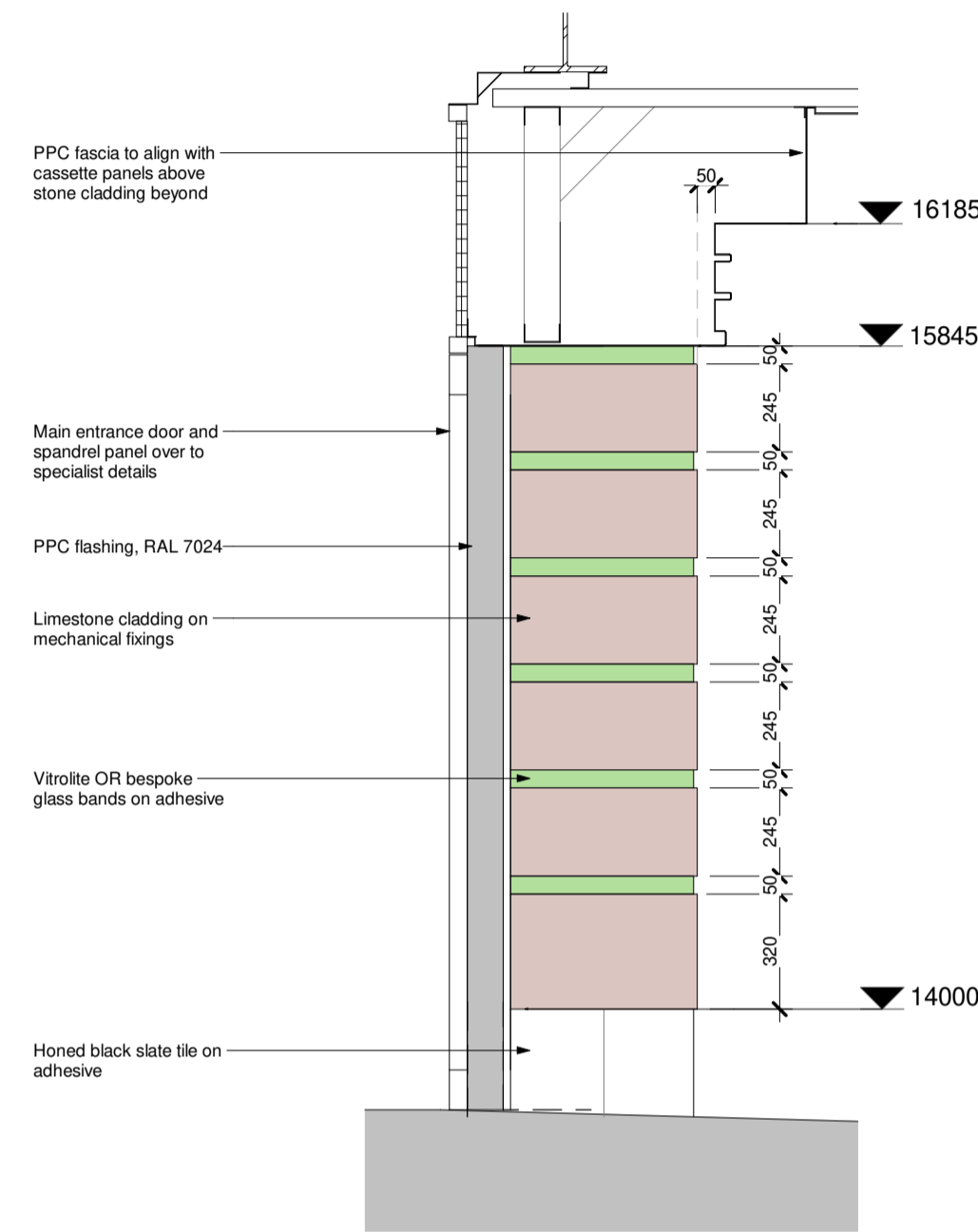
Elev A 1 : 20
