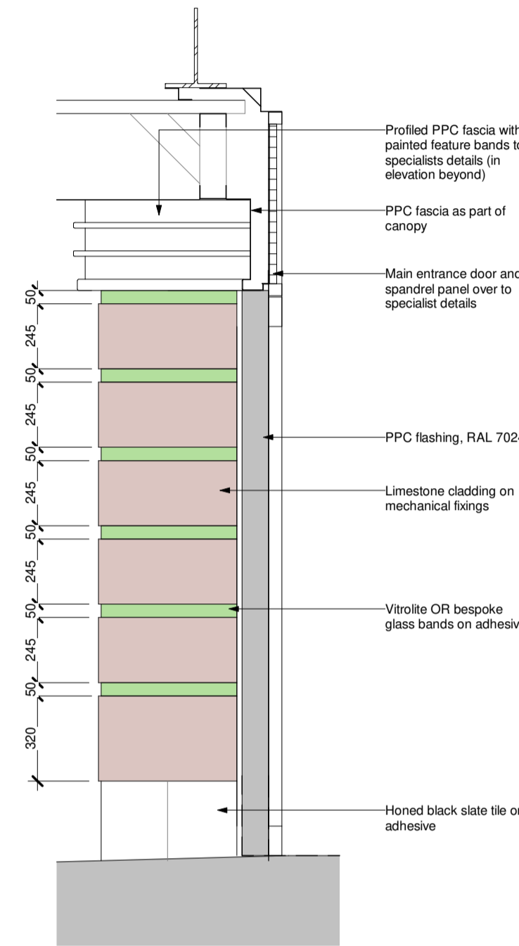
Elev C
