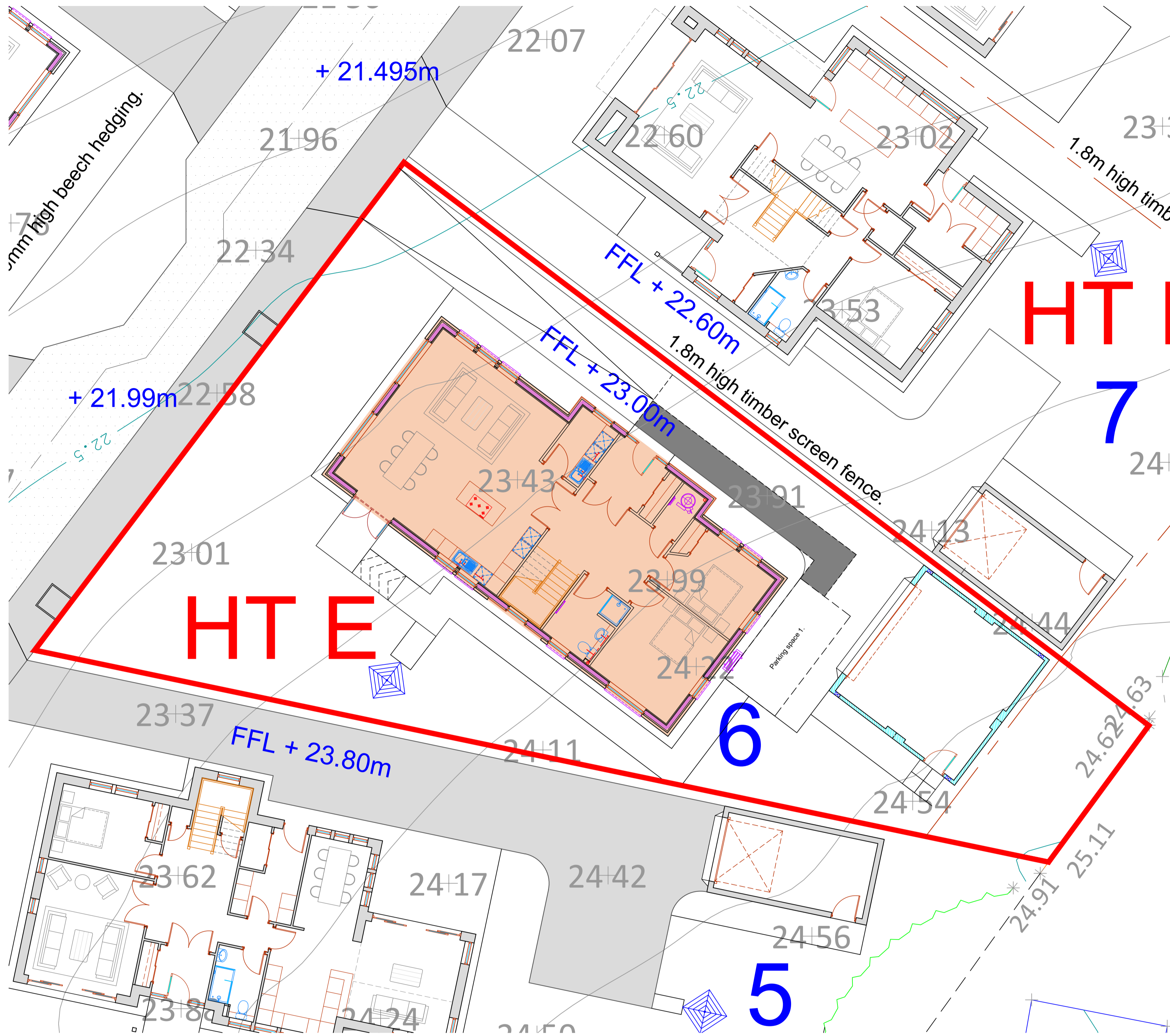
Site plan 1:100
