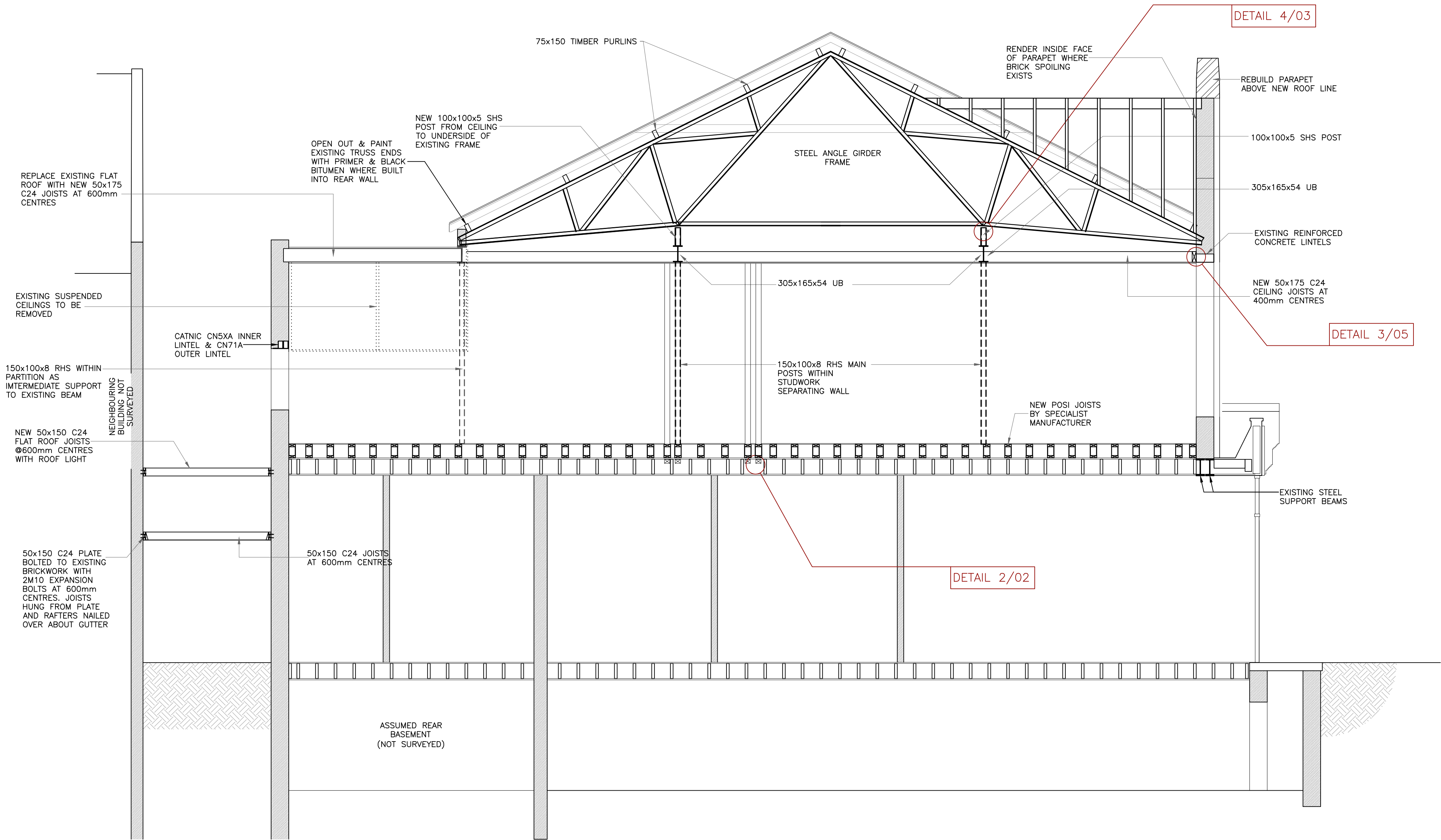
SECTION A-A 1:50
