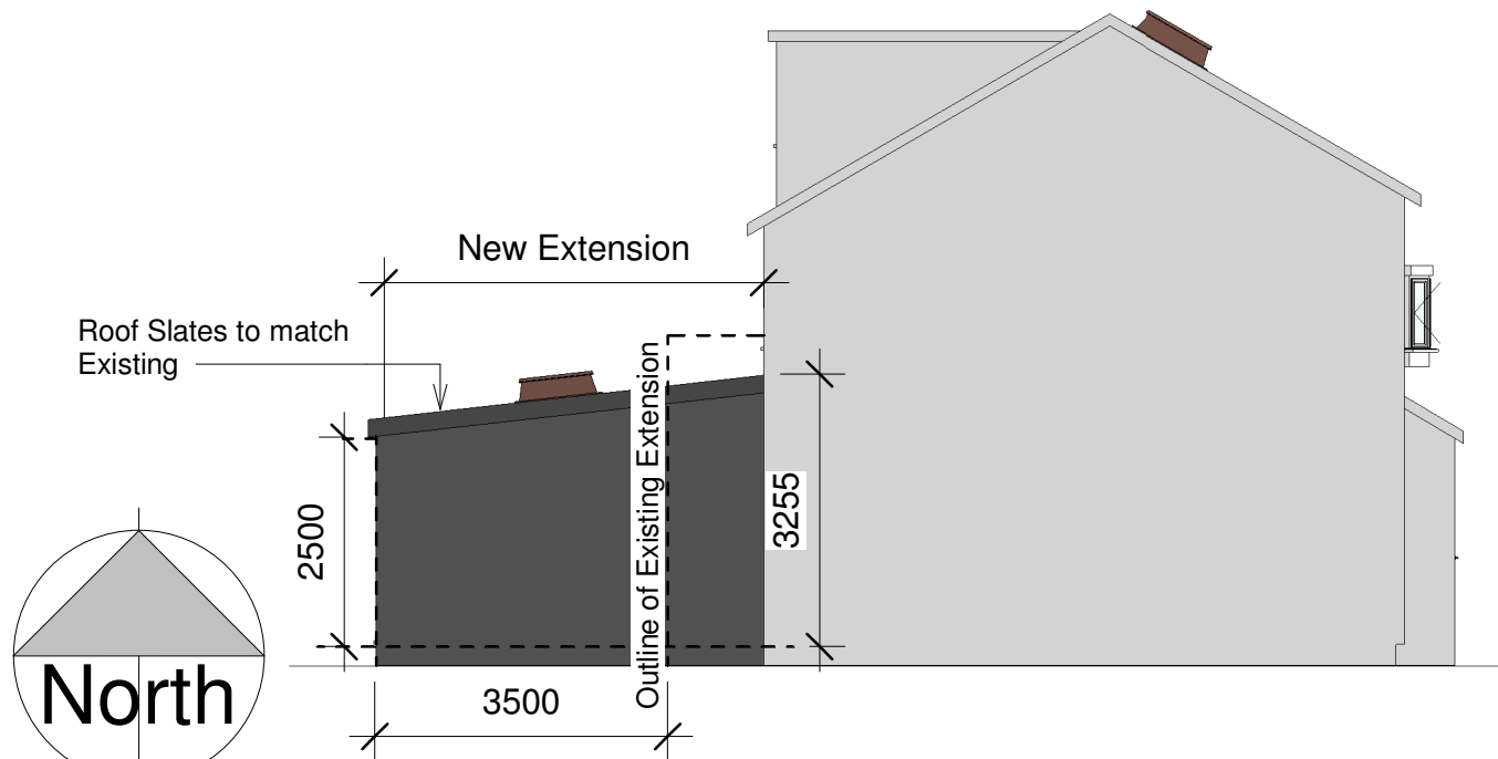
3 Elevation 3 - a 1 : 100
