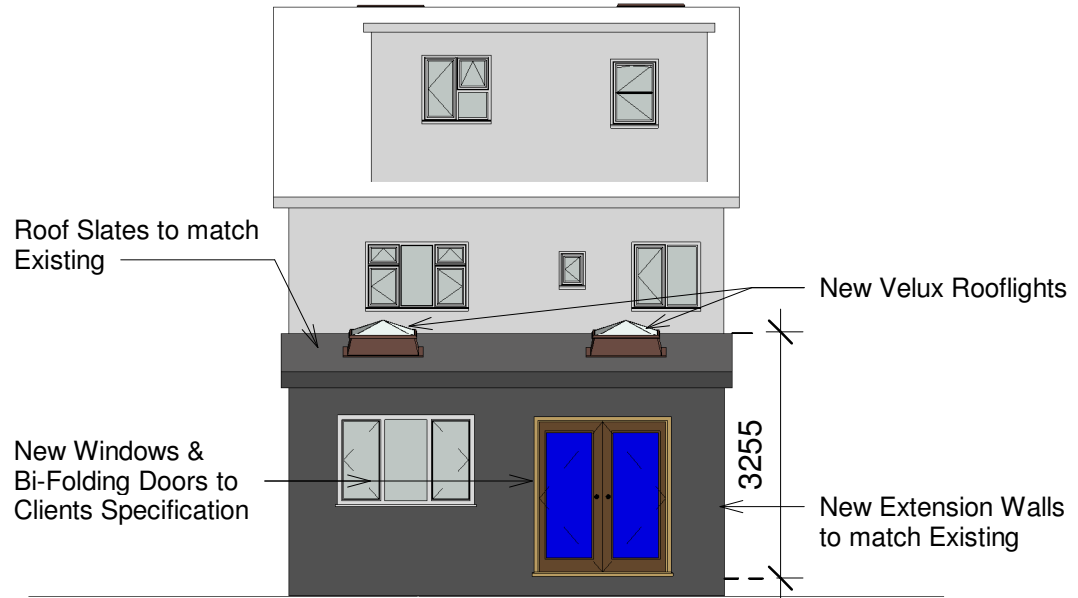
2 Elevation 2 - a 1 : 100
