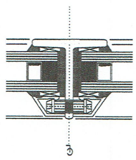
GLAZING BAR
