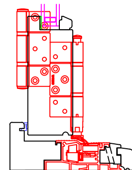
Door Cill
