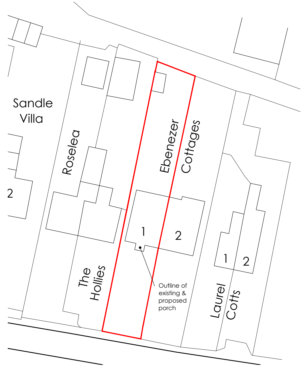
2 Site Plan 1 : 500
