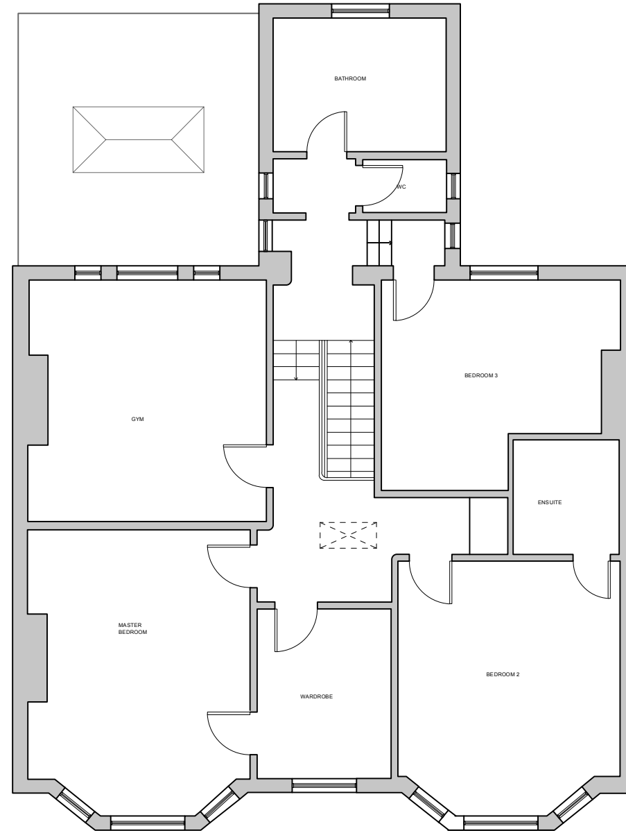
2 First Floor Scale: 1:100
