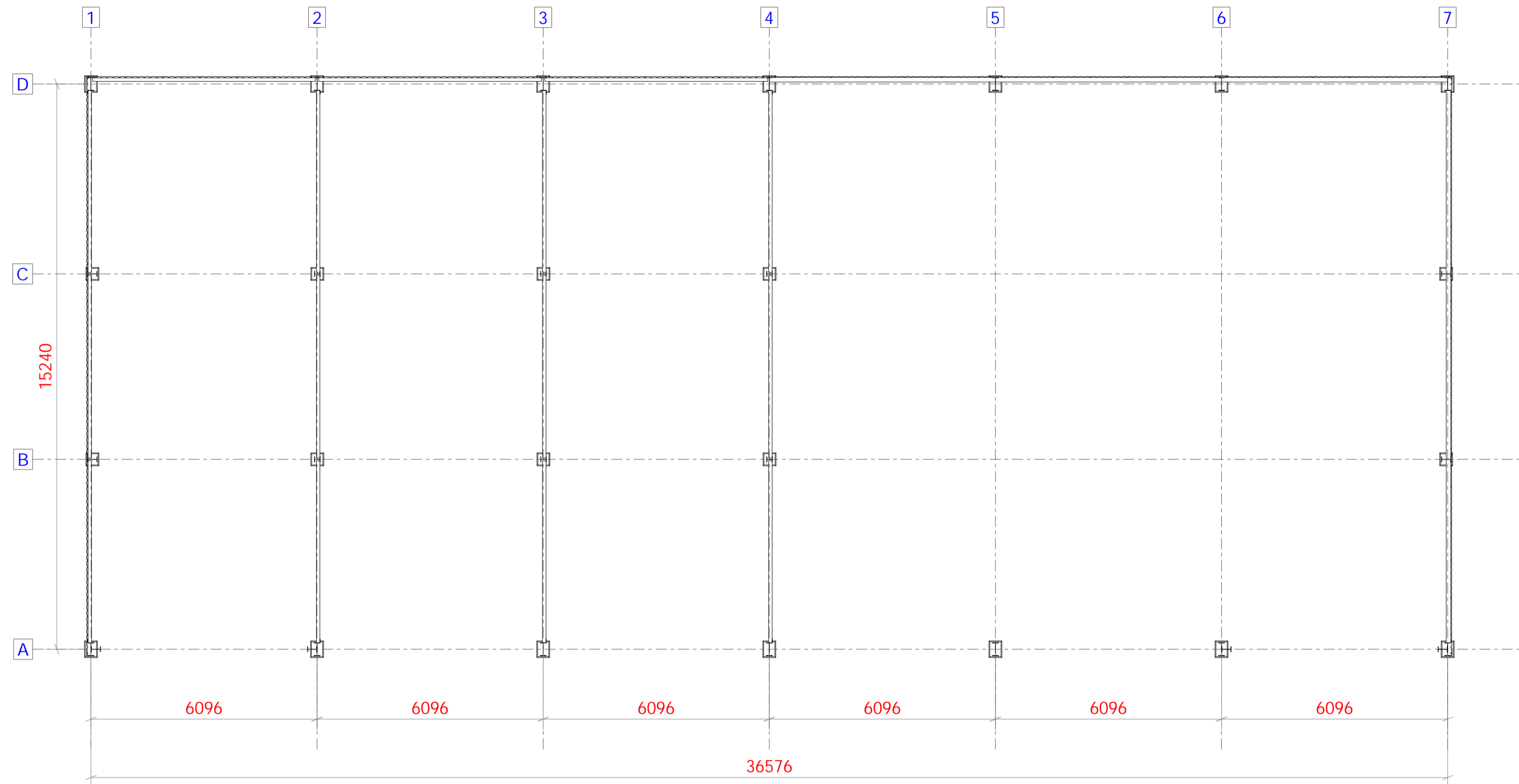
Plan FFL
