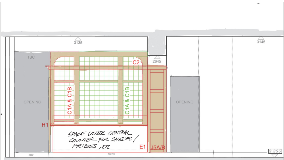
SECTION D-D
