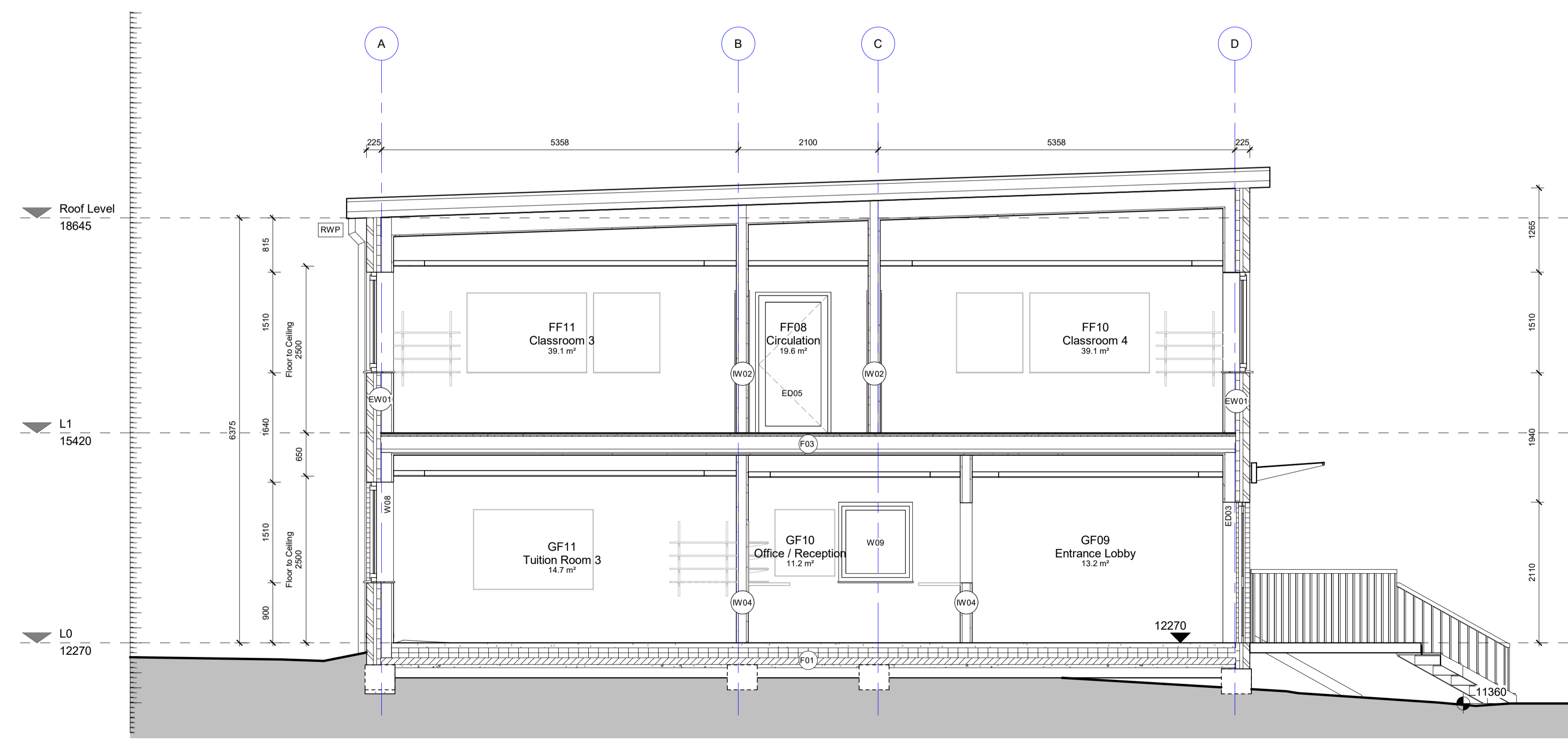
Section BB 1 : 50
