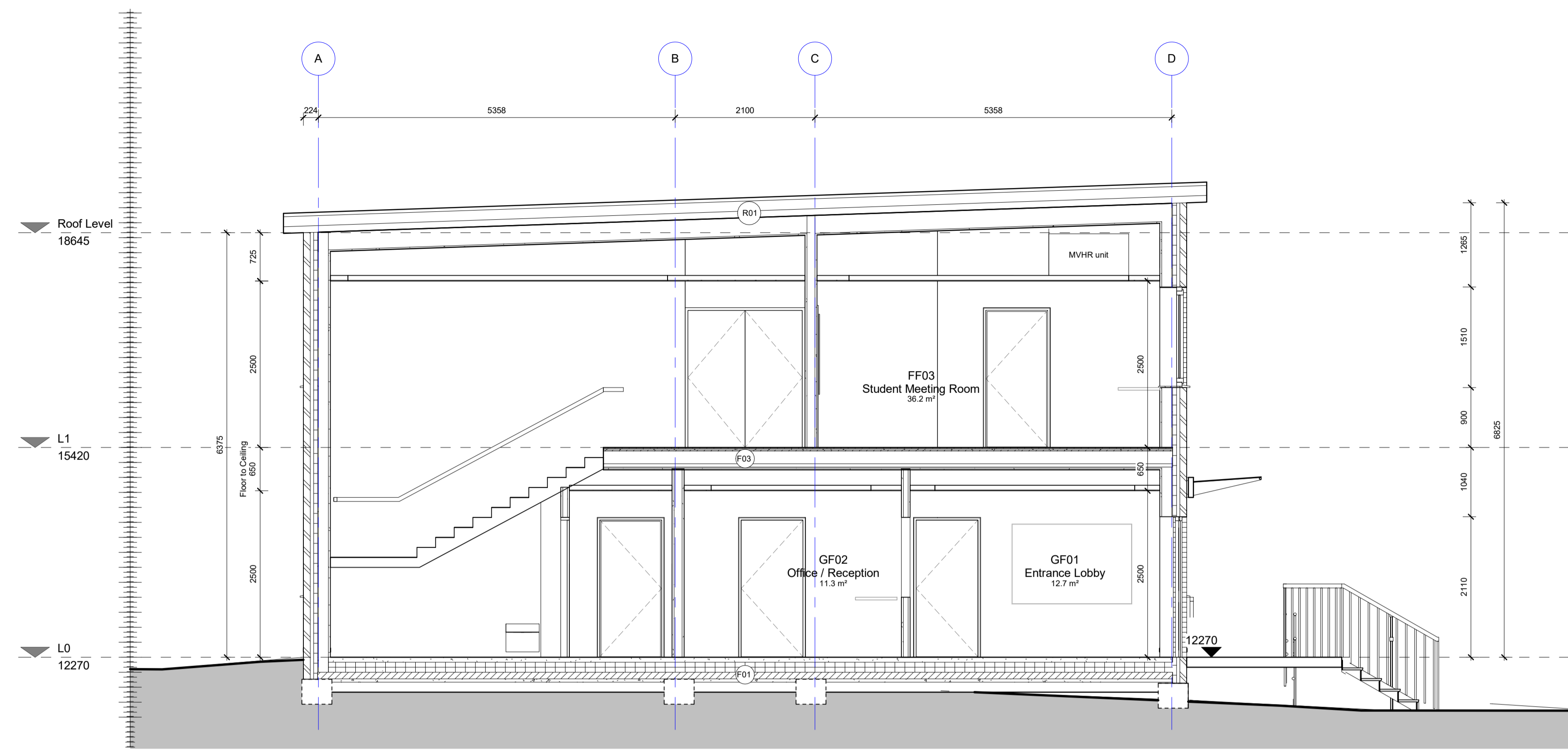
Section AA 1 : 50
