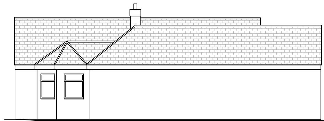
RIGHT ELEVATION
