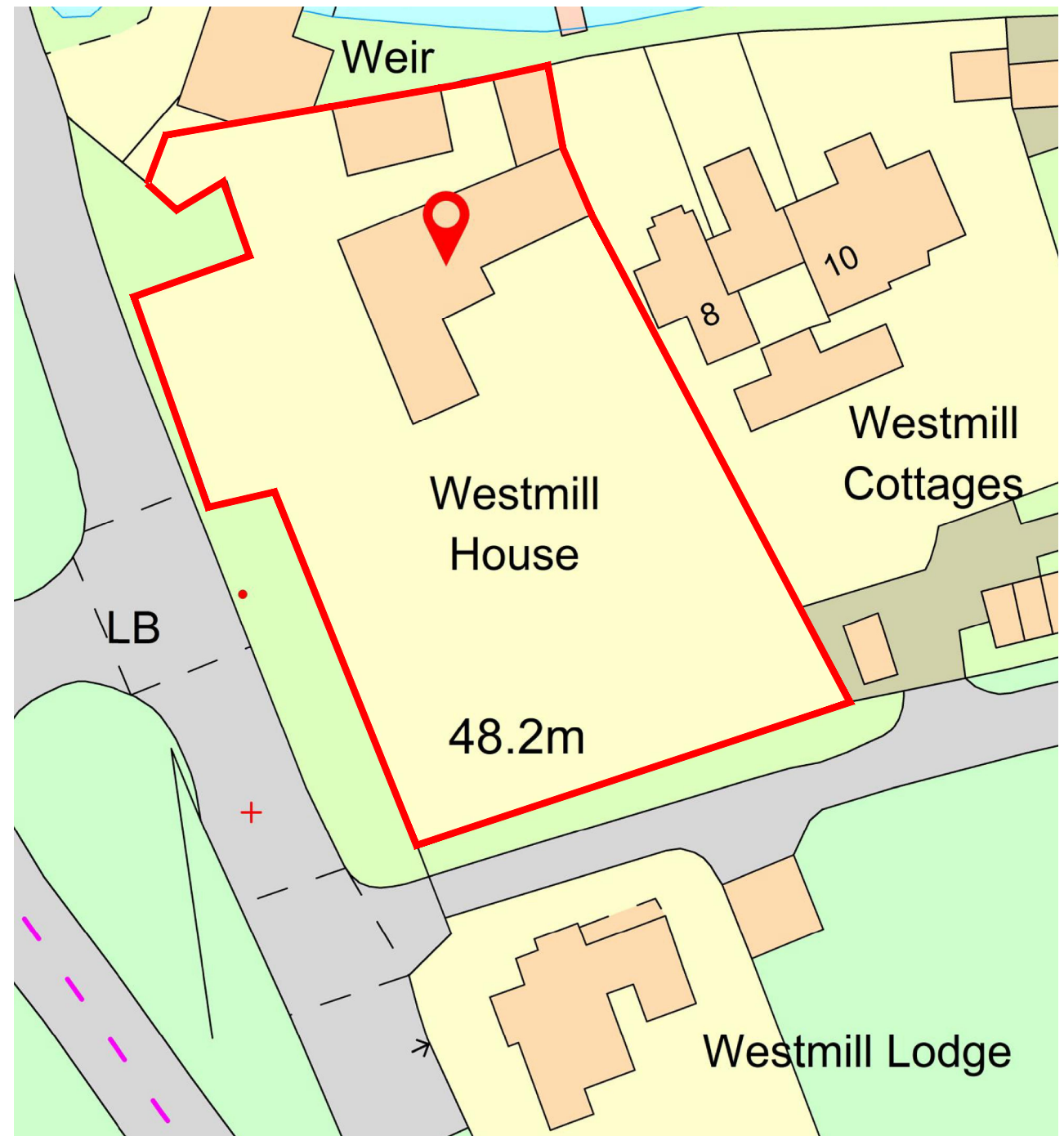
2 Site Plan 1:500
