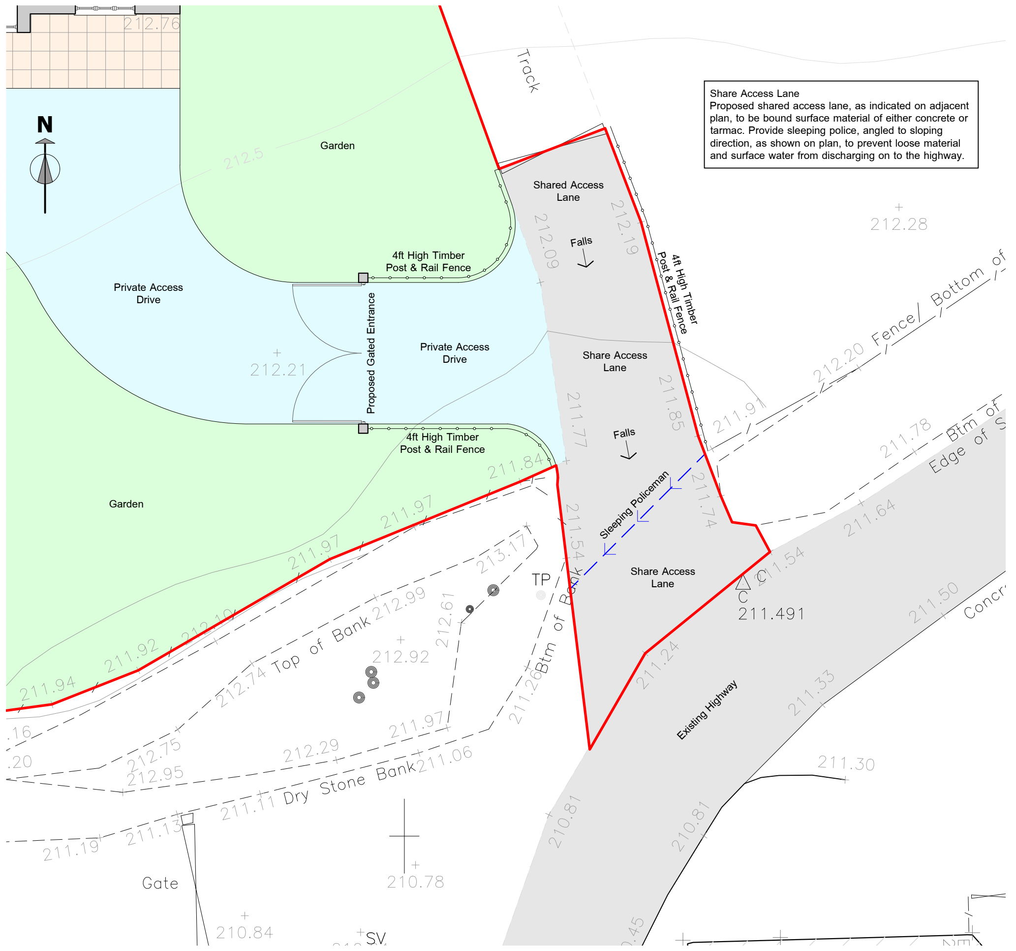
Part Site Plan 1:100
