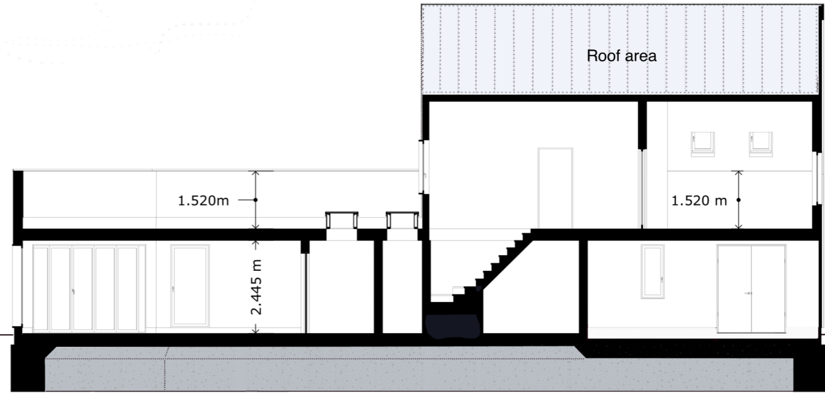
Section E1, Drawing PLNG / 02 / 10 A
