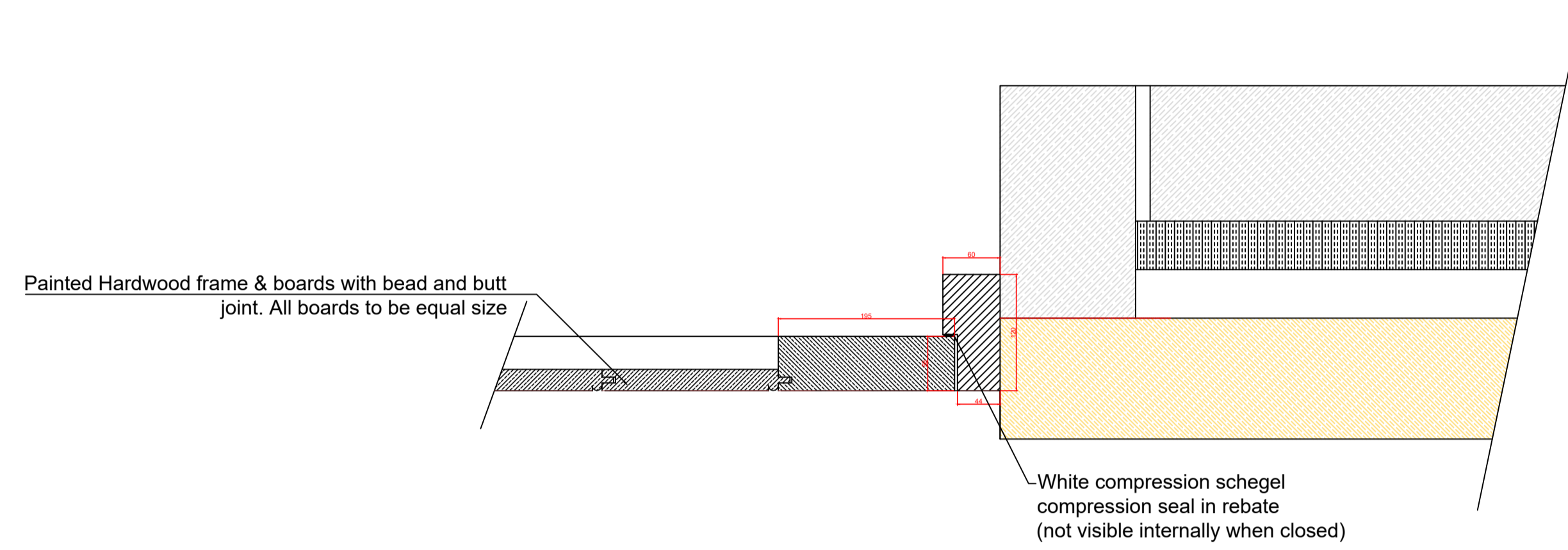
C-C DOOR JAMB SECTION
