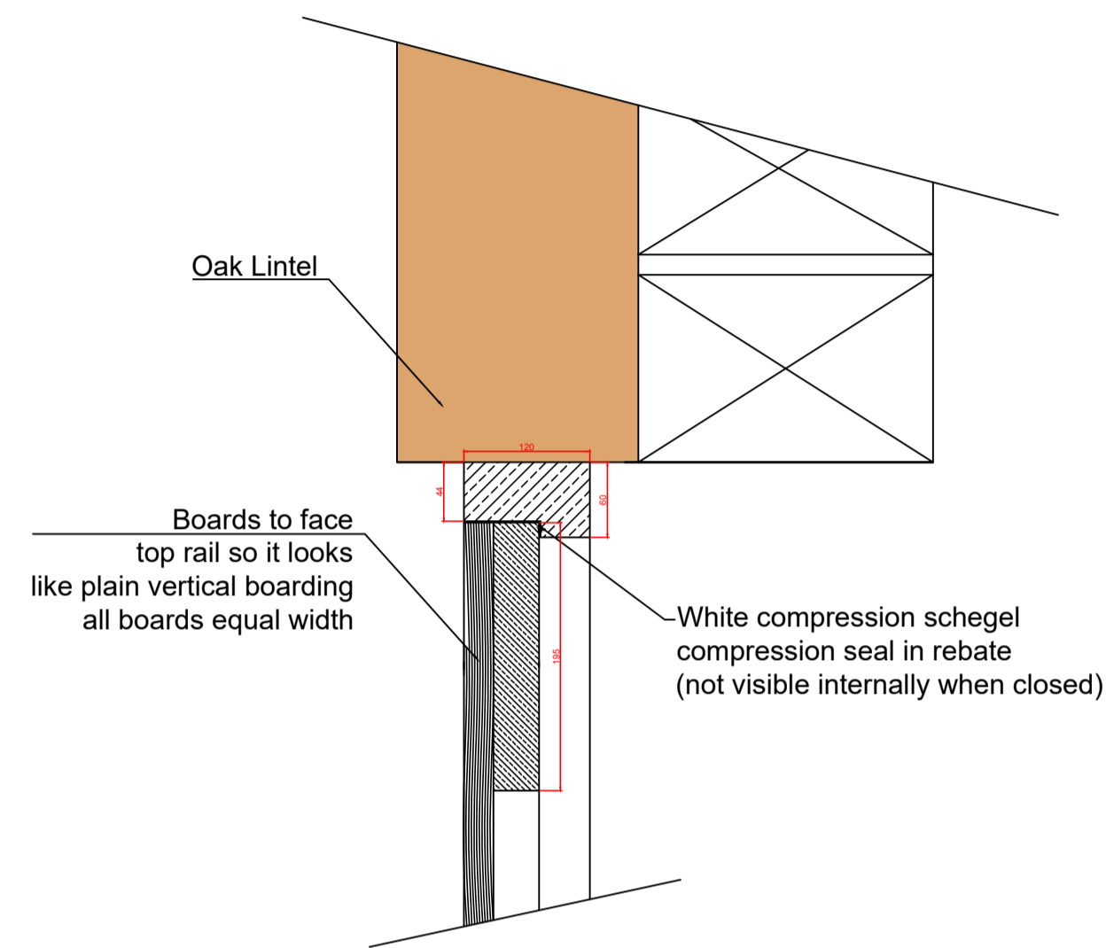
A-A DOOR HEAD SECTION
