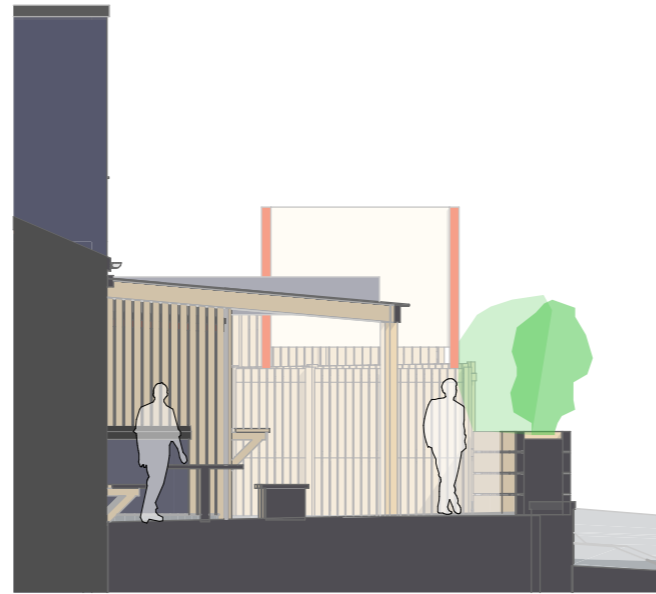
Section S3.1 1:100
