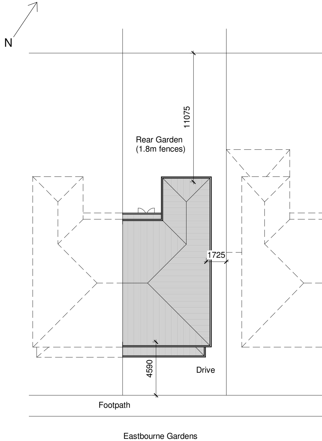
1 Site 1 : 200
